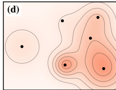
CIOC [Levine '12]
