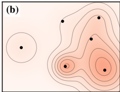
Implicit (ours)
