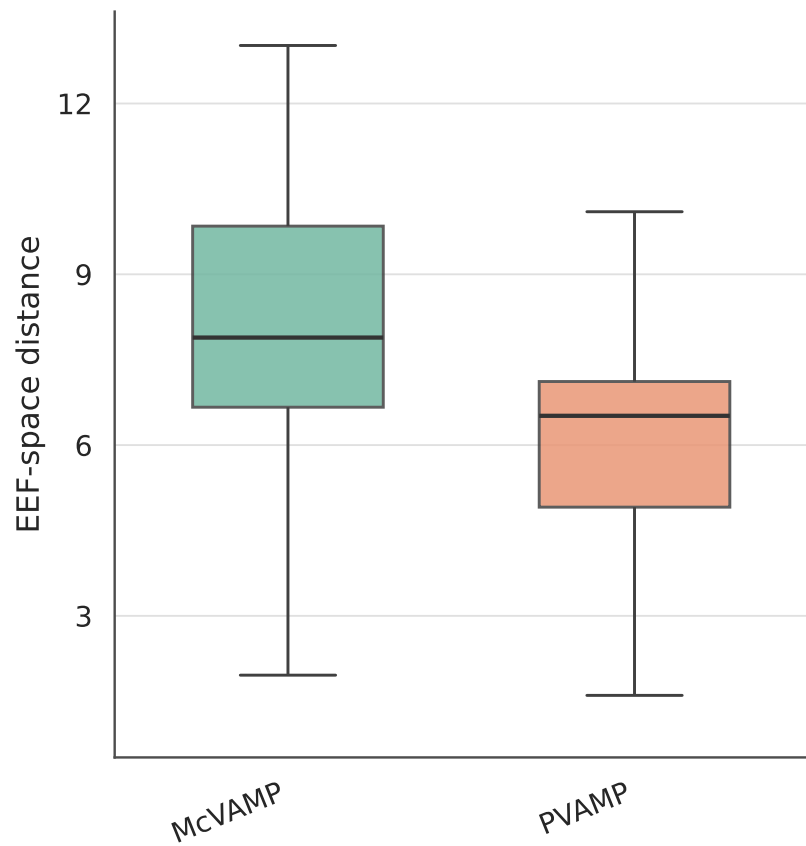
EEF-space distance
