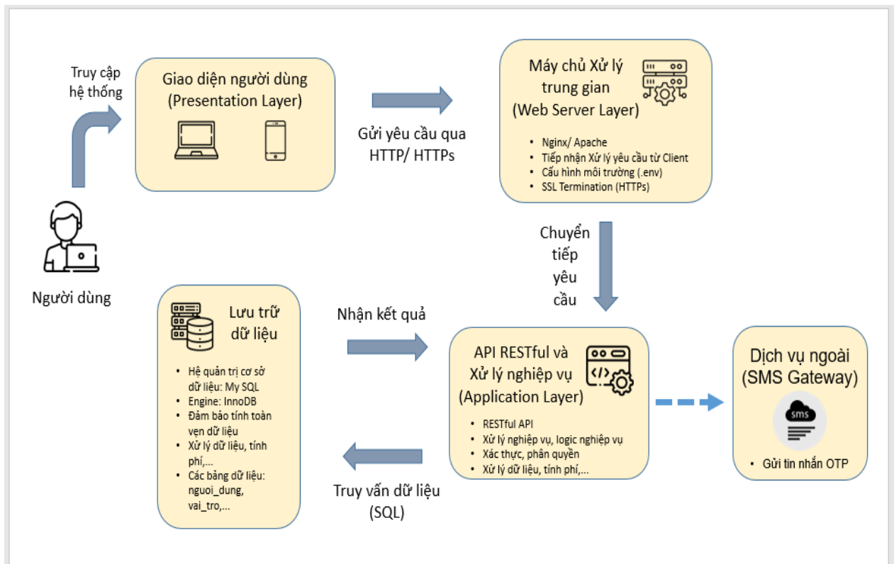
Hình 3.1. Sơ đồ kiến trúc hệ thống
