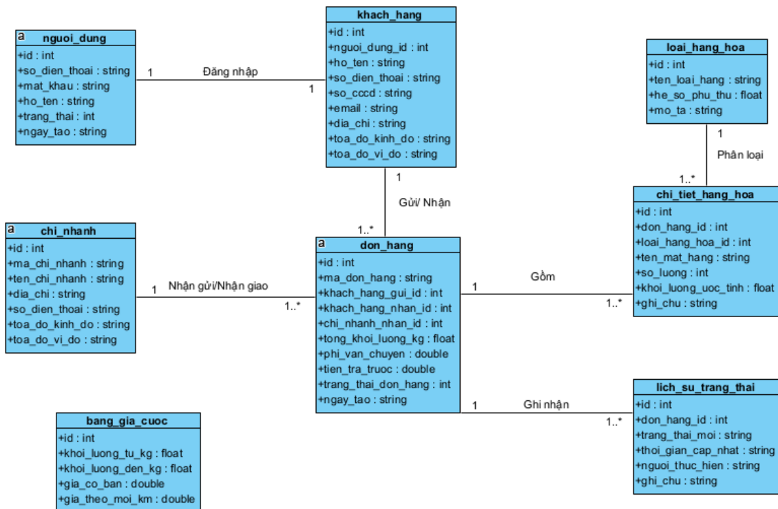
Hình 3.5. Lược đồ nhóm khách hàng và đơn hàng
