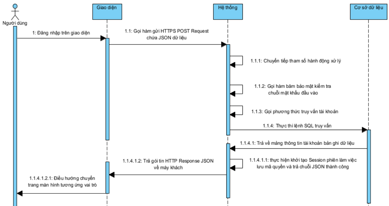
Hình 3.17. Sơ đồ tuần tự Đăng nhập hệ thống
