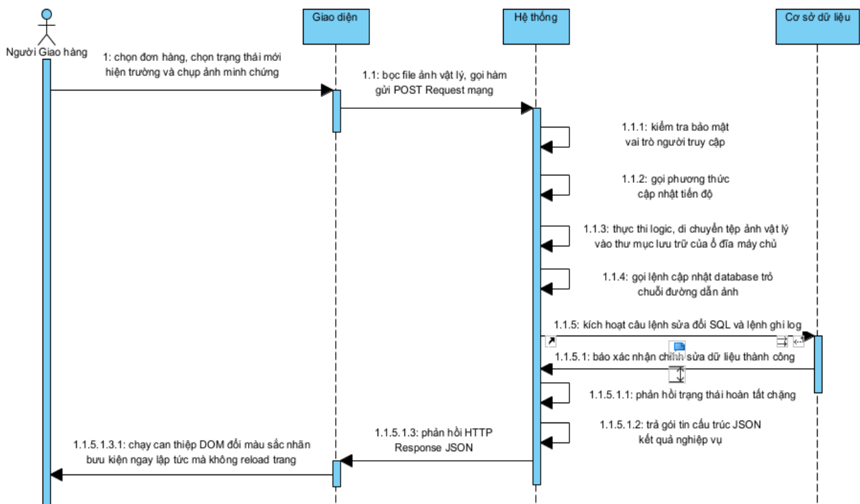
Hình 3.19. Sơ đồ tuần tự Cập nhật tiến độ giao hàng
