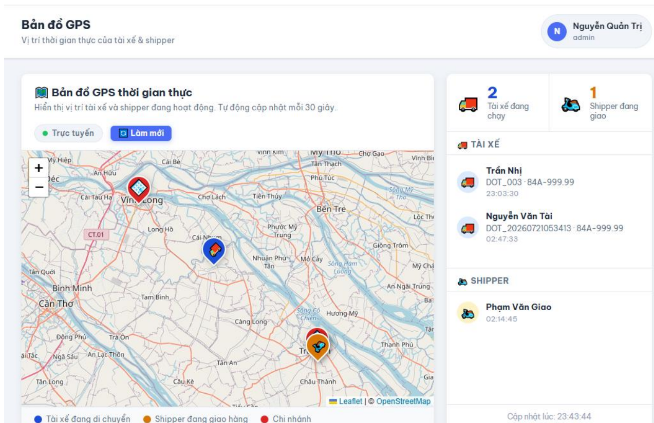
Hình 4.13. Giao diện Bản đồ GPS
