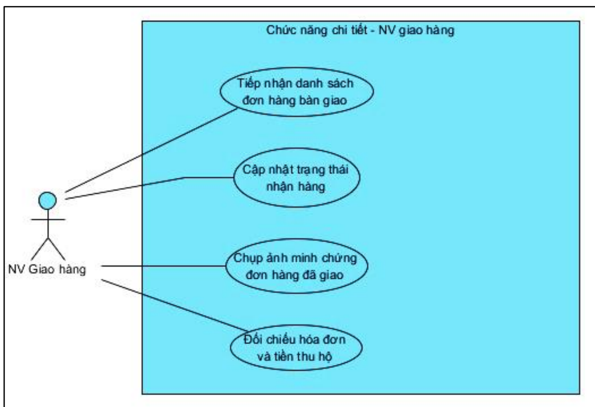
Hình 3.12. Sơ đồ use case người giao hàng
