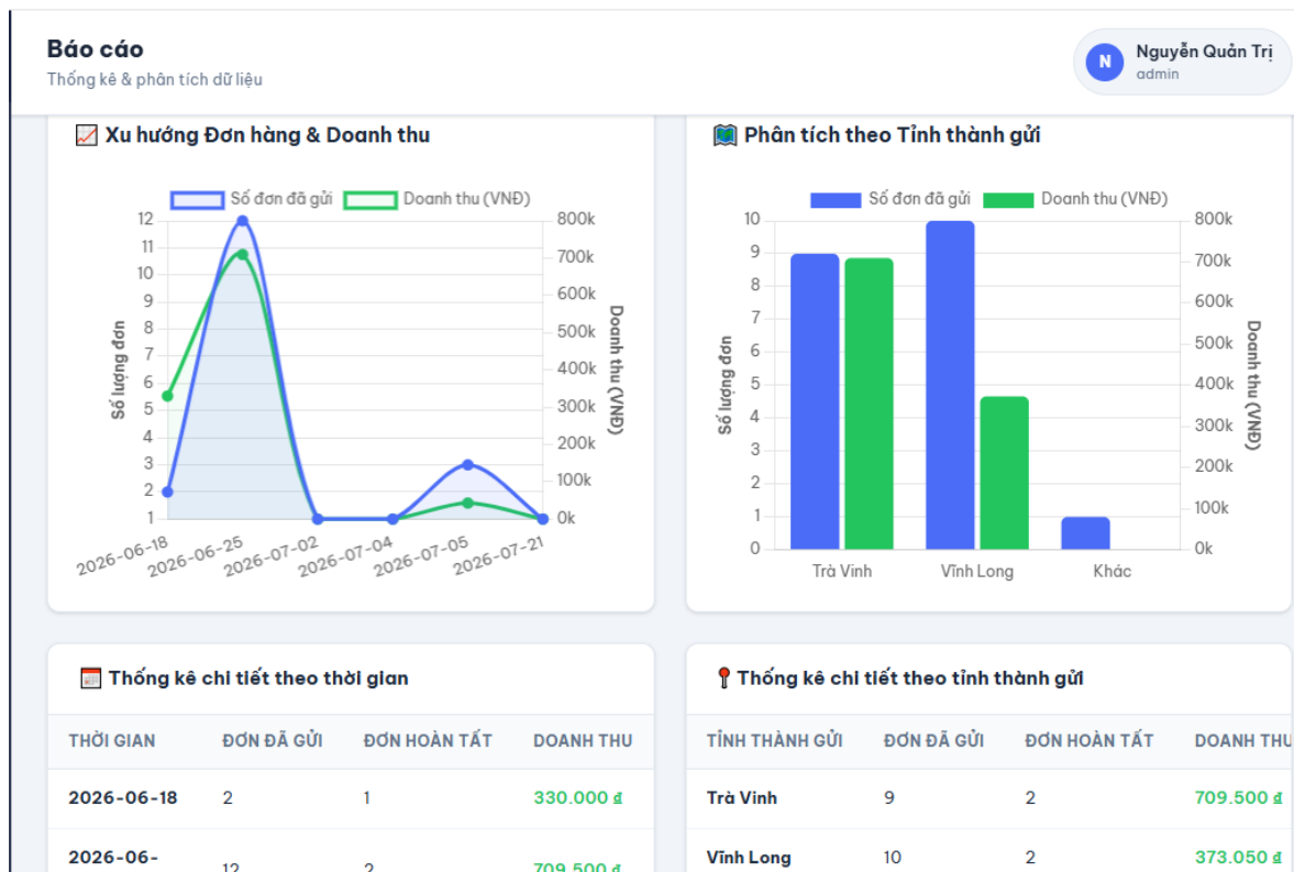
Hình 4.15. Giao diện trang báo cáo thống kê 2
