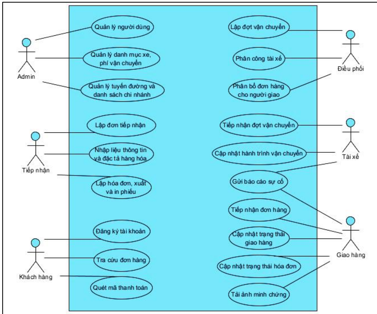
Hình 3.7. Sơ đồ use case tổng quát
