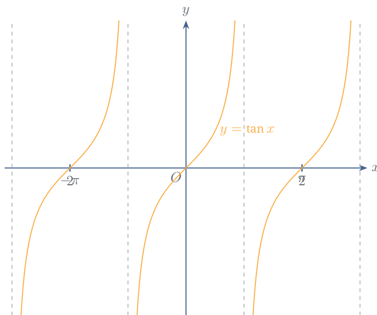
图 3: 正切函数图像
