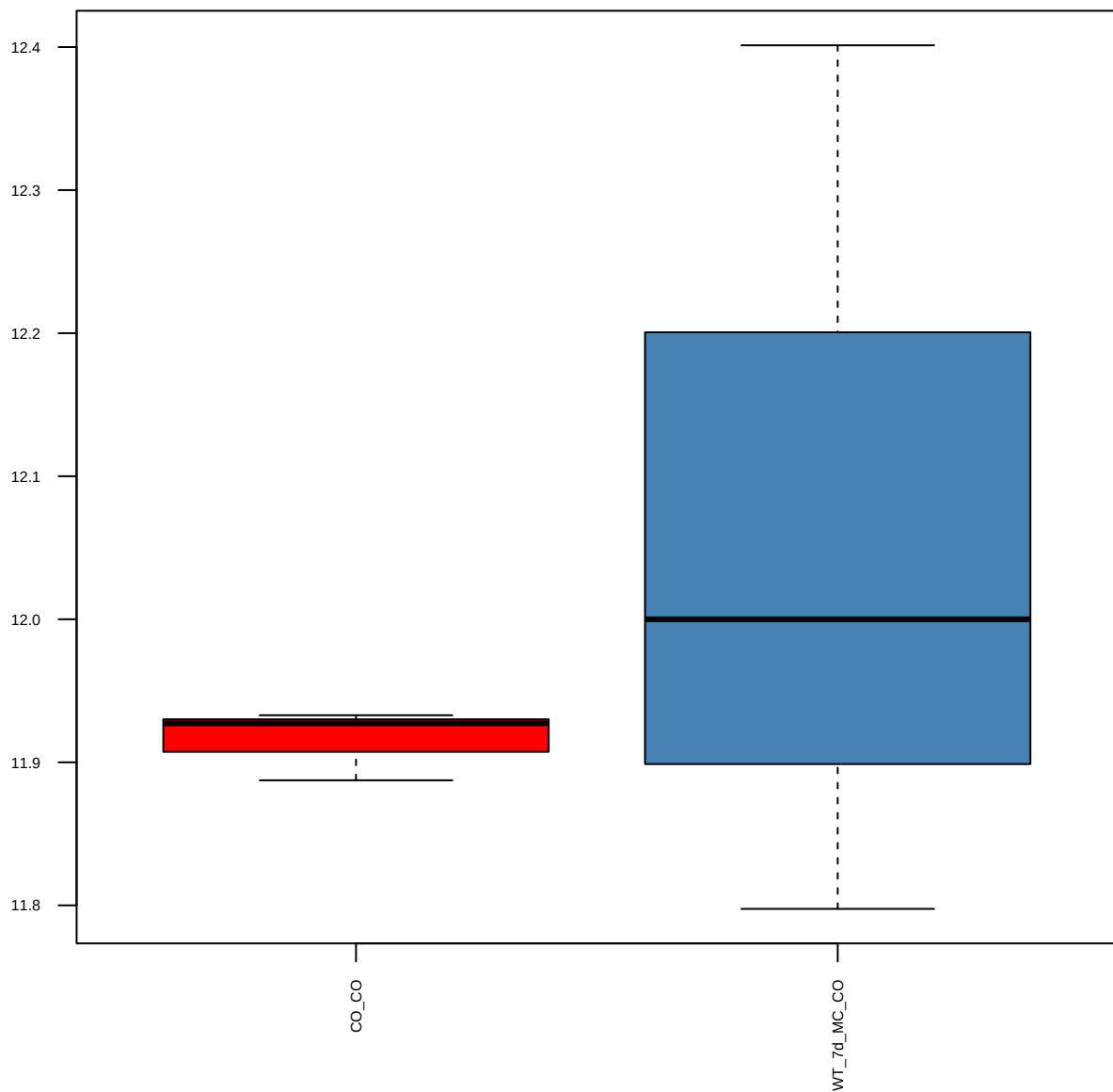
MED12-Abcam (FDR = 0.9)
