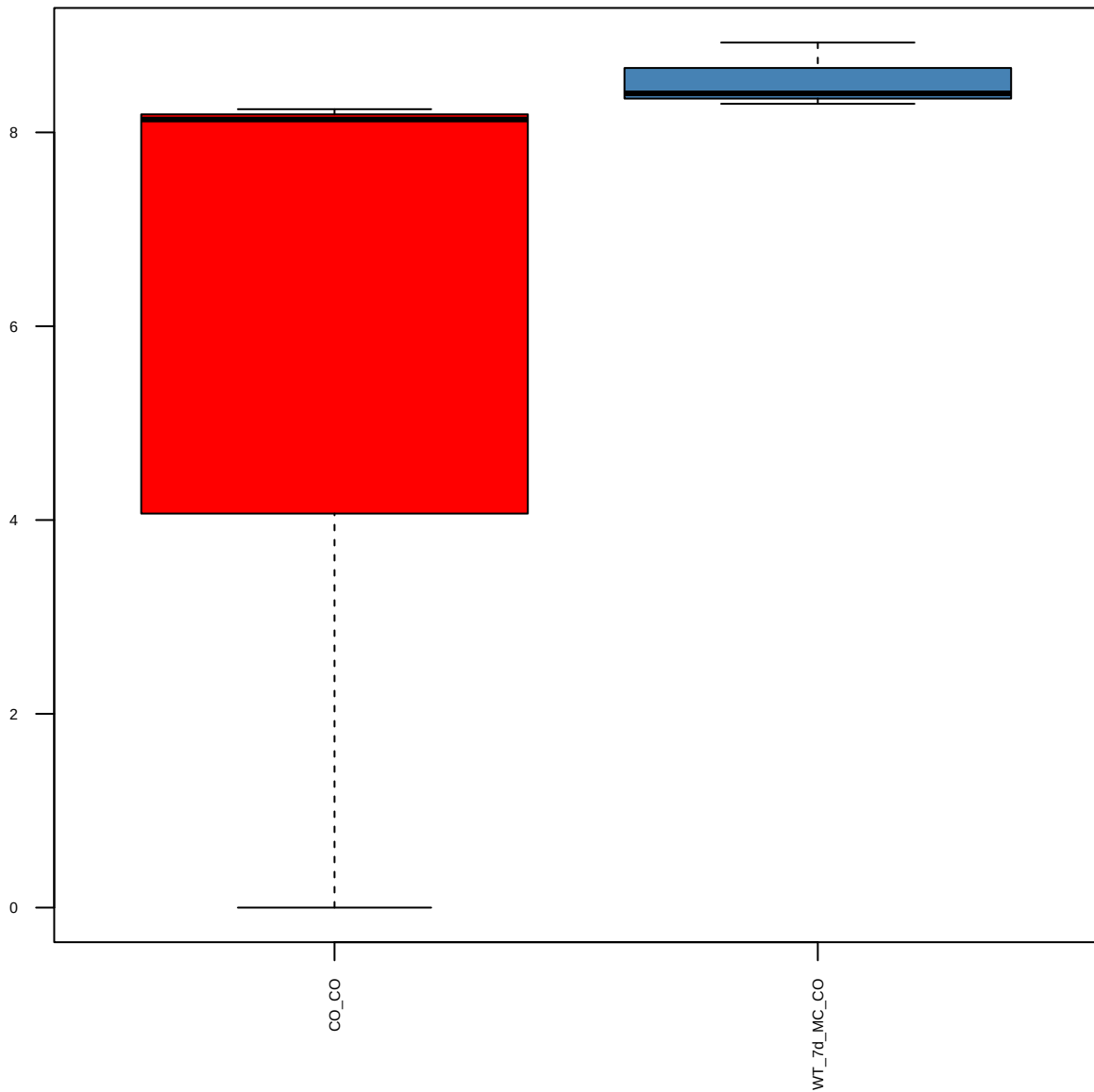
p27/KIP1(C-term) (FDR = 0.9)
