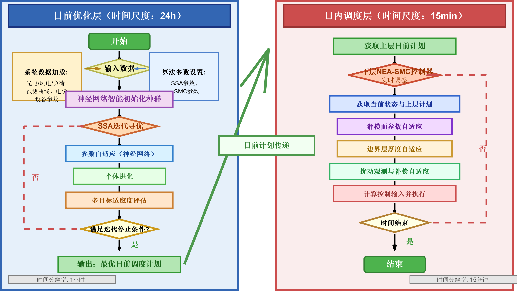
多时间尺度双层优化调度框架
