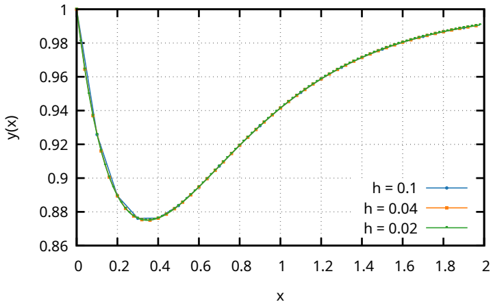
Solución RK4 con distintos pasos h
