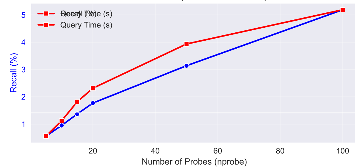
Recall vs Query Time - llama-128-ip
