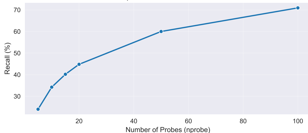
Recall vs nprobe - llama-128-ip
