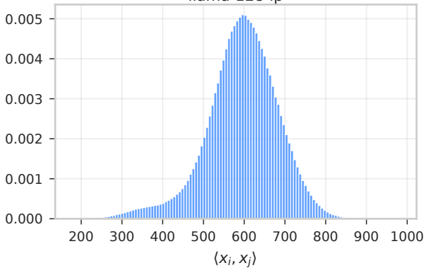
llama-128-ip
