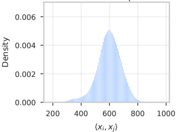
llama-128-ip
