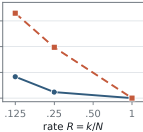
DocVQA
