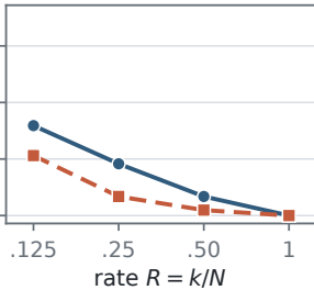
GQA
