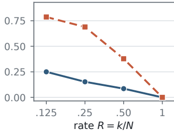
TextVQA
