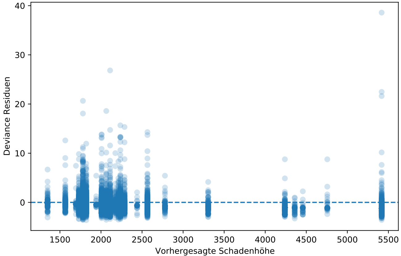
Deviance-Residuen vs. vorhergesagte Severity
