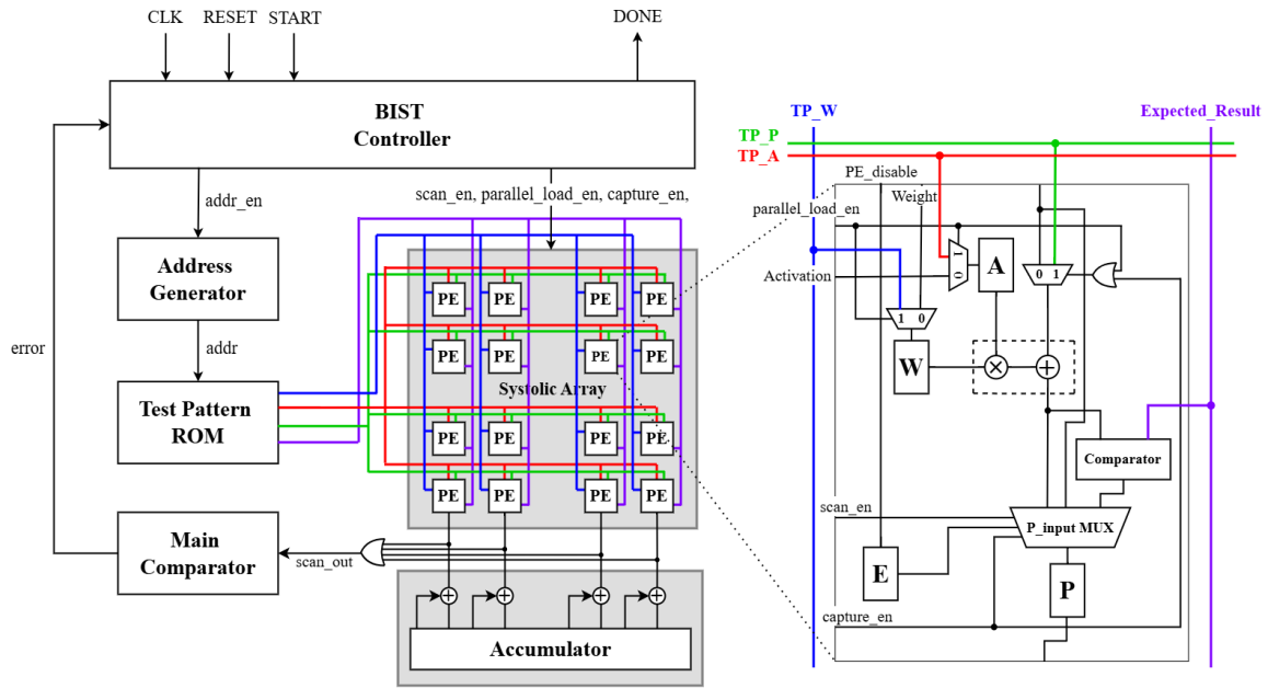
그림 3. BICS-BIST의 구성 모듈 및 자가 진단 구조
