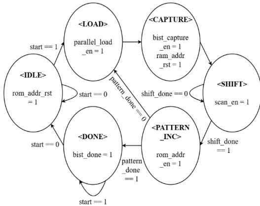
그림 2. BICS-BIST Controller 의 FSM 다이어그램
