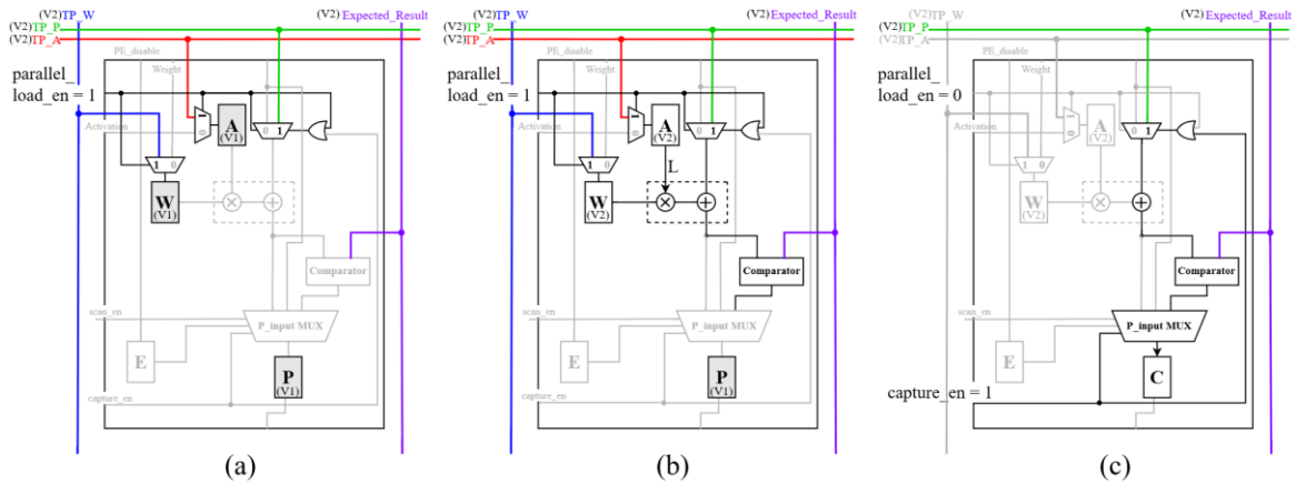
그림 5. BICS-BIST의 TD 테스트 (a) 초기화, (b) 런치 이벤트, (c) At-speed 캡처
