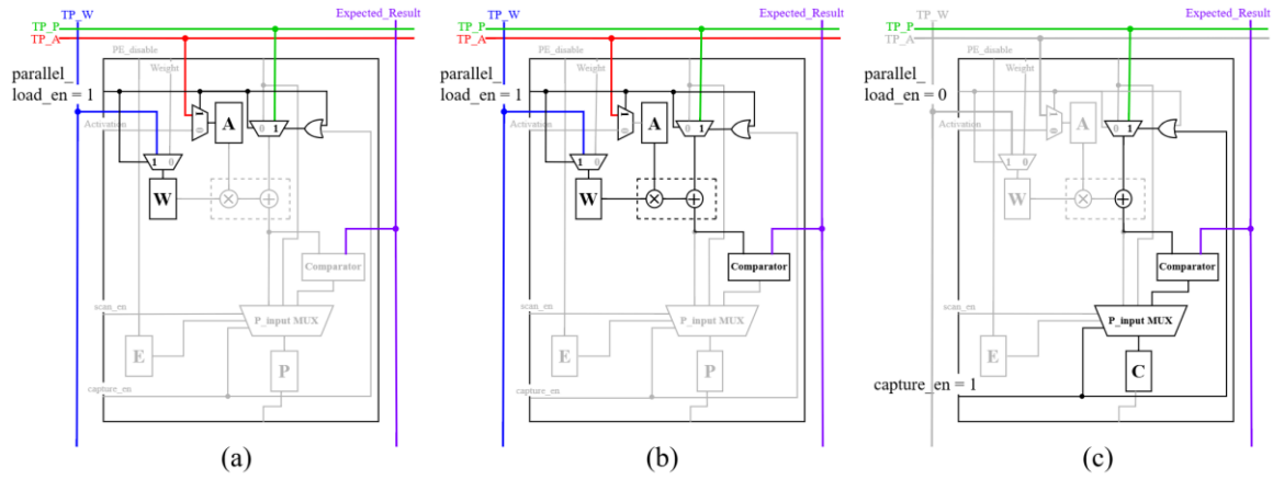
그림 4. BICS-BIST의 SA 테스트 (a) 병렬 패턴 로드, (b) 연산 및 비교, (c) 결과 캡처
