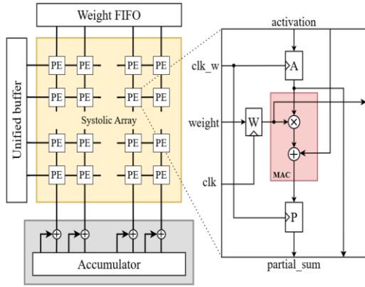
그림 1. Systolic Array-based AI 가속기 구조
