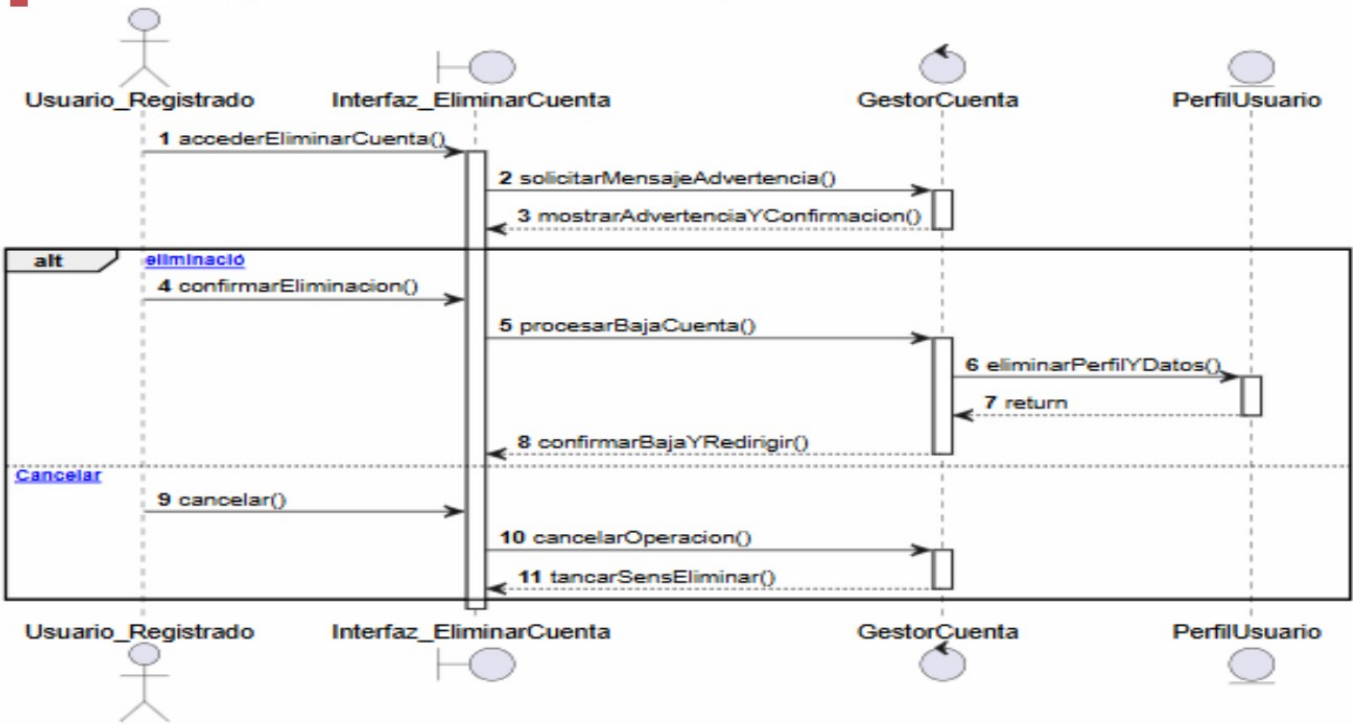
Figura 11. Diagrama de seqüència - Eliminar Compte.
