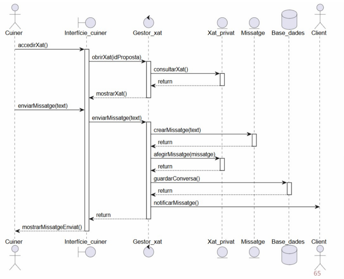
Figura 28. Diagrama de seqüència - Comunicar-se amb el client mitjançant xat privat.
