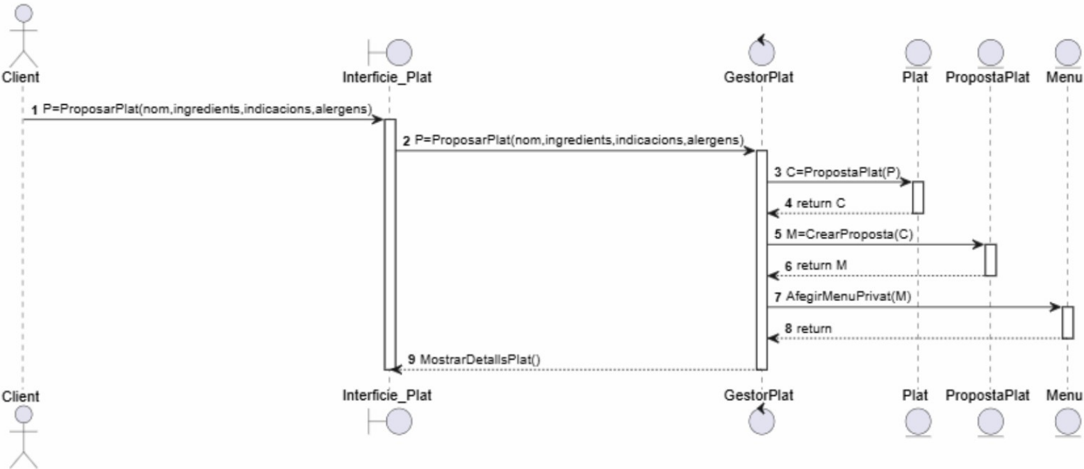
Figura 17. Diagrama de seqüència - Proposar plat.
