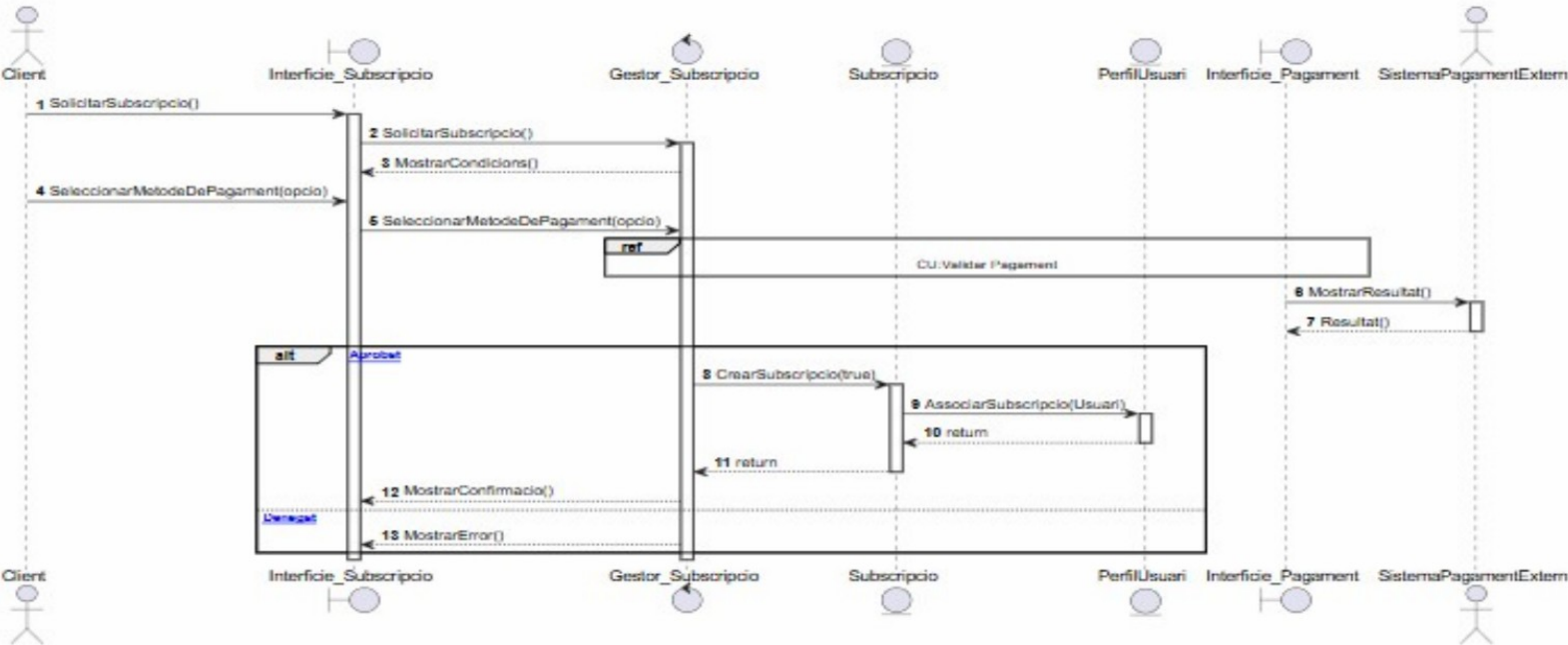
Figura 23. Diagrama de seqüència - Subscriure's al pla mensual.
