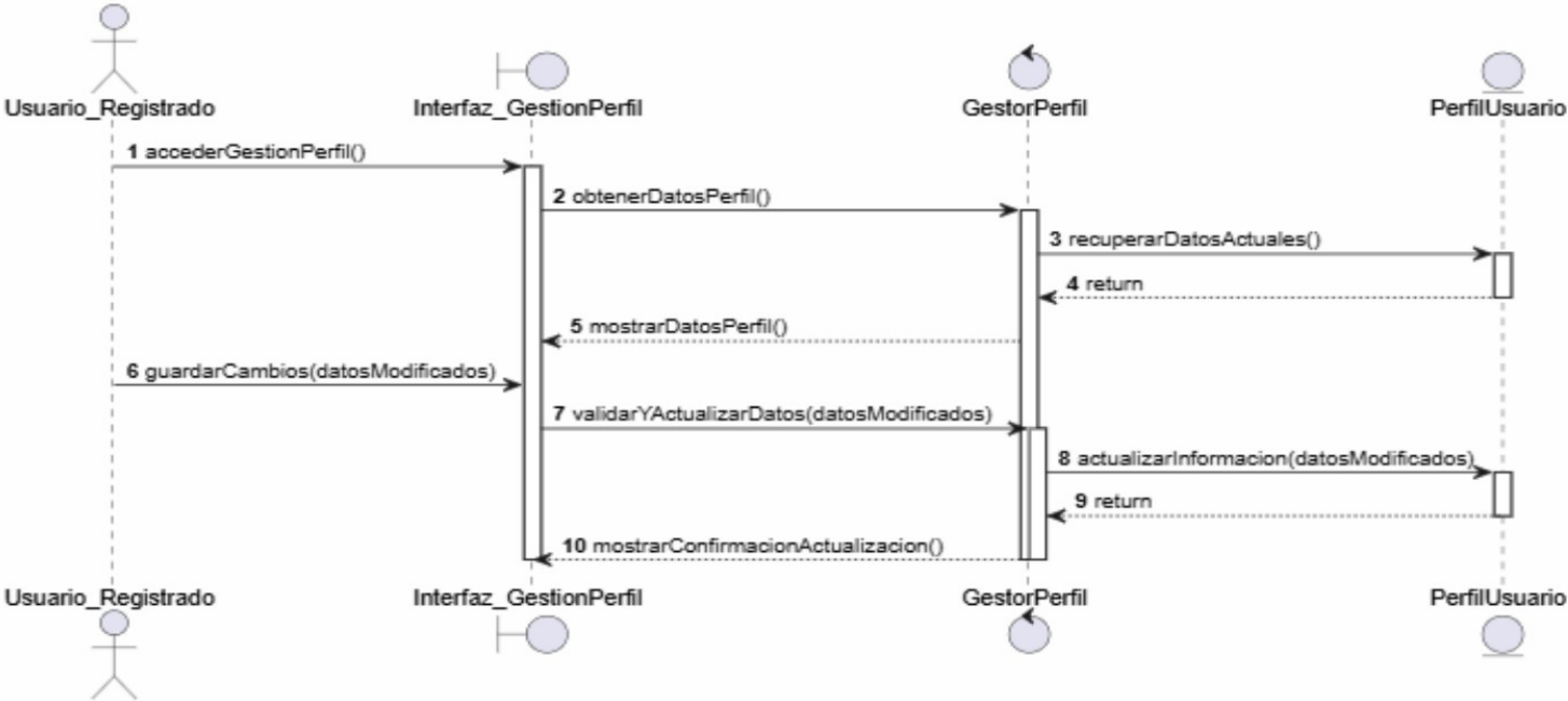
Figura 10. Diagrama de seqüència - Gestionar Perfil.
