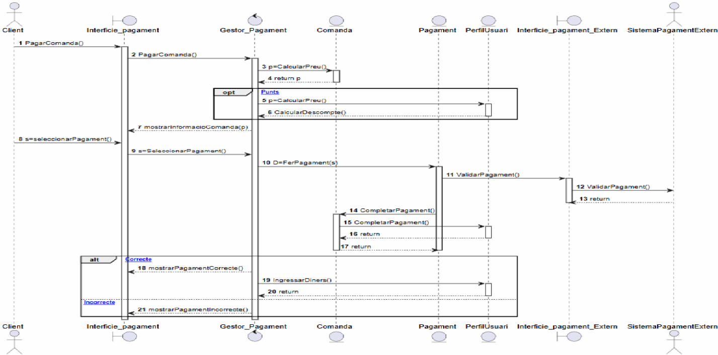
Figura 14. Diagrama de seqüència - Pagar comanda.
