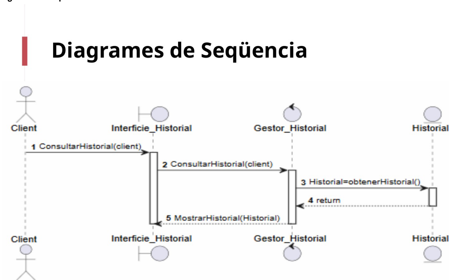
Figura 21. Diagrama de seqüència - Consultar historial de comandes.
