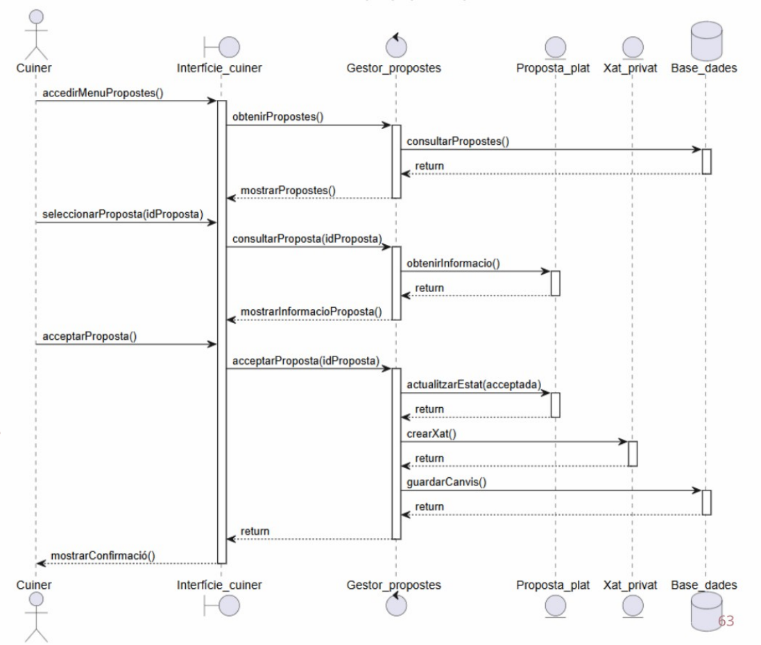
Figura 27. Diagrama de seqüència - Acceptar proposta de plat.
