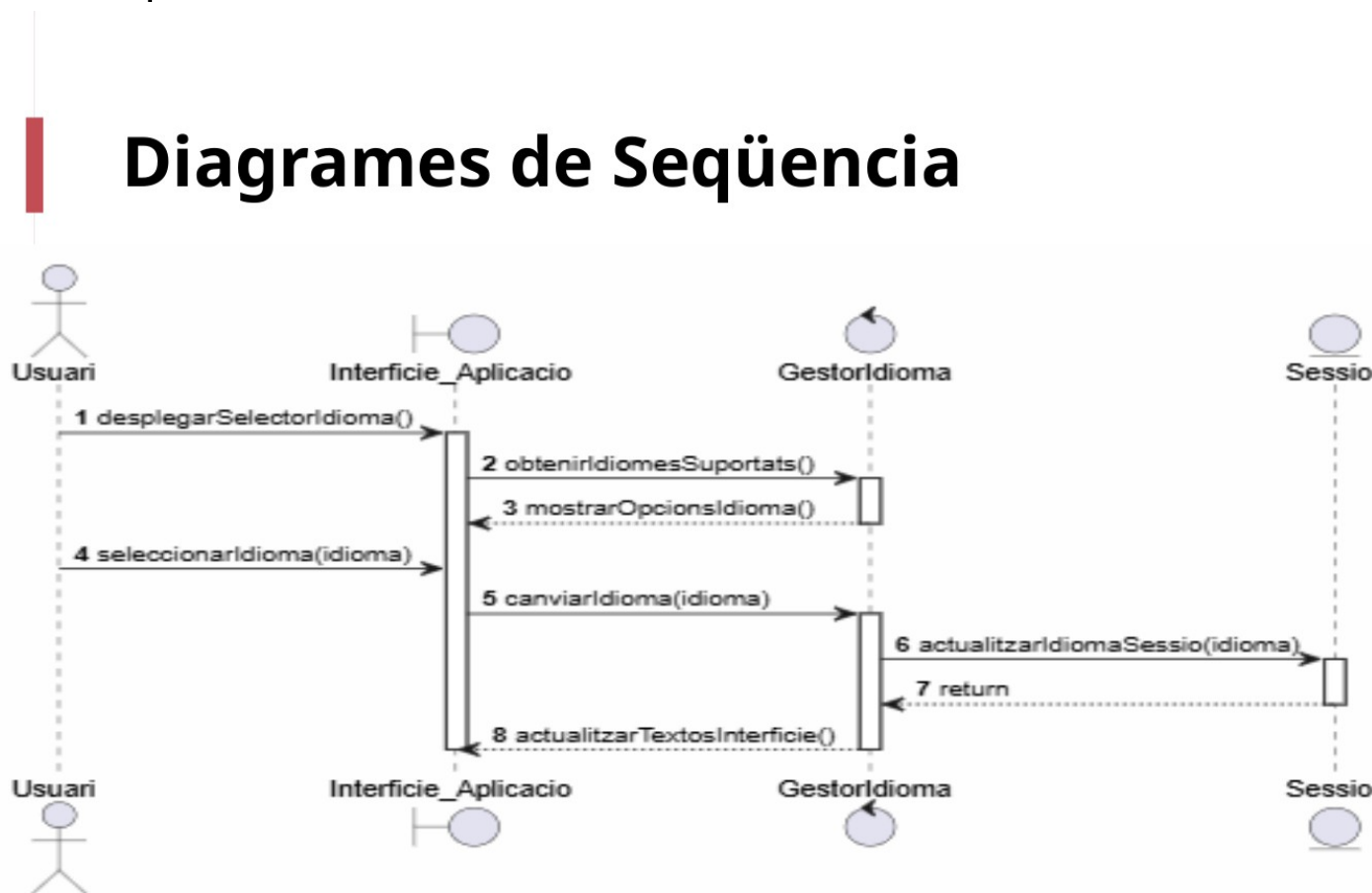
Figura 13. Diagrama de seqüència - Canviar idioma.
