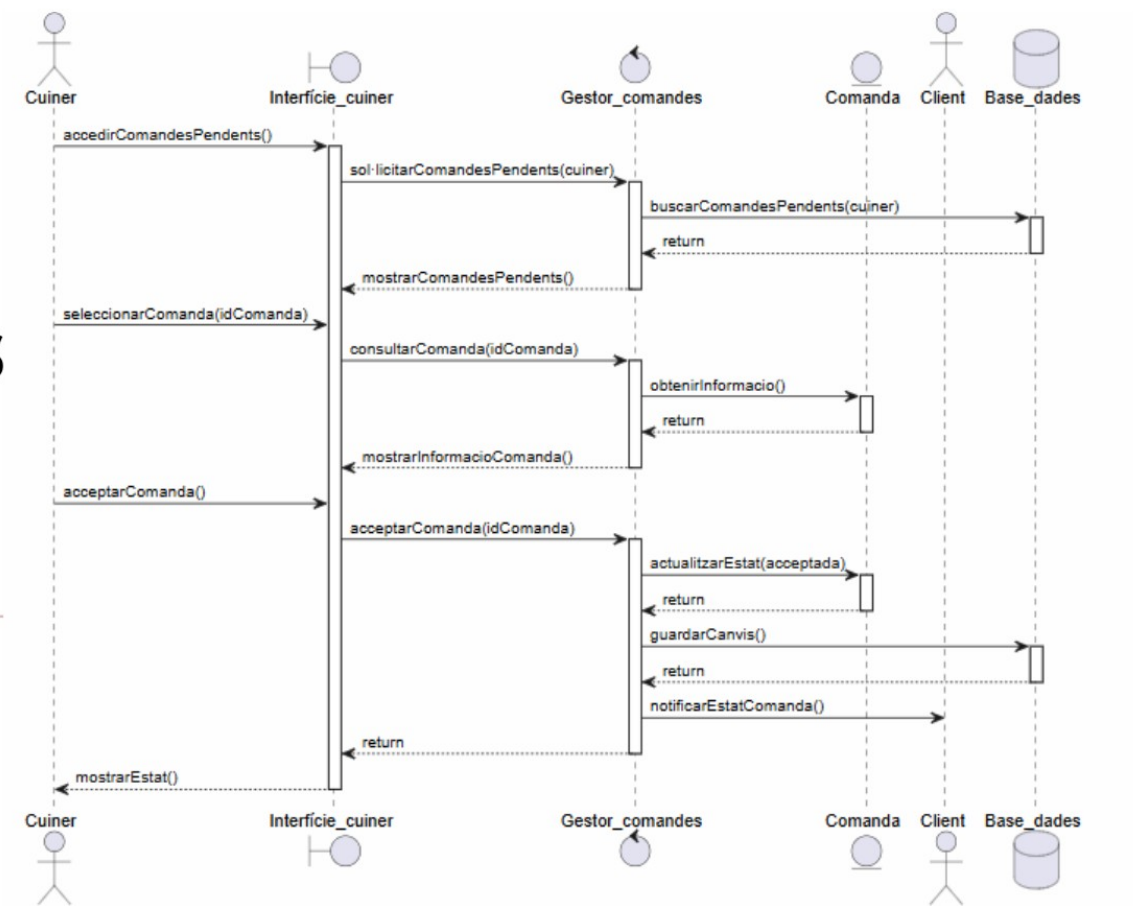
Figura 26. Diagrama de seqüència - Acceptar comandes.
