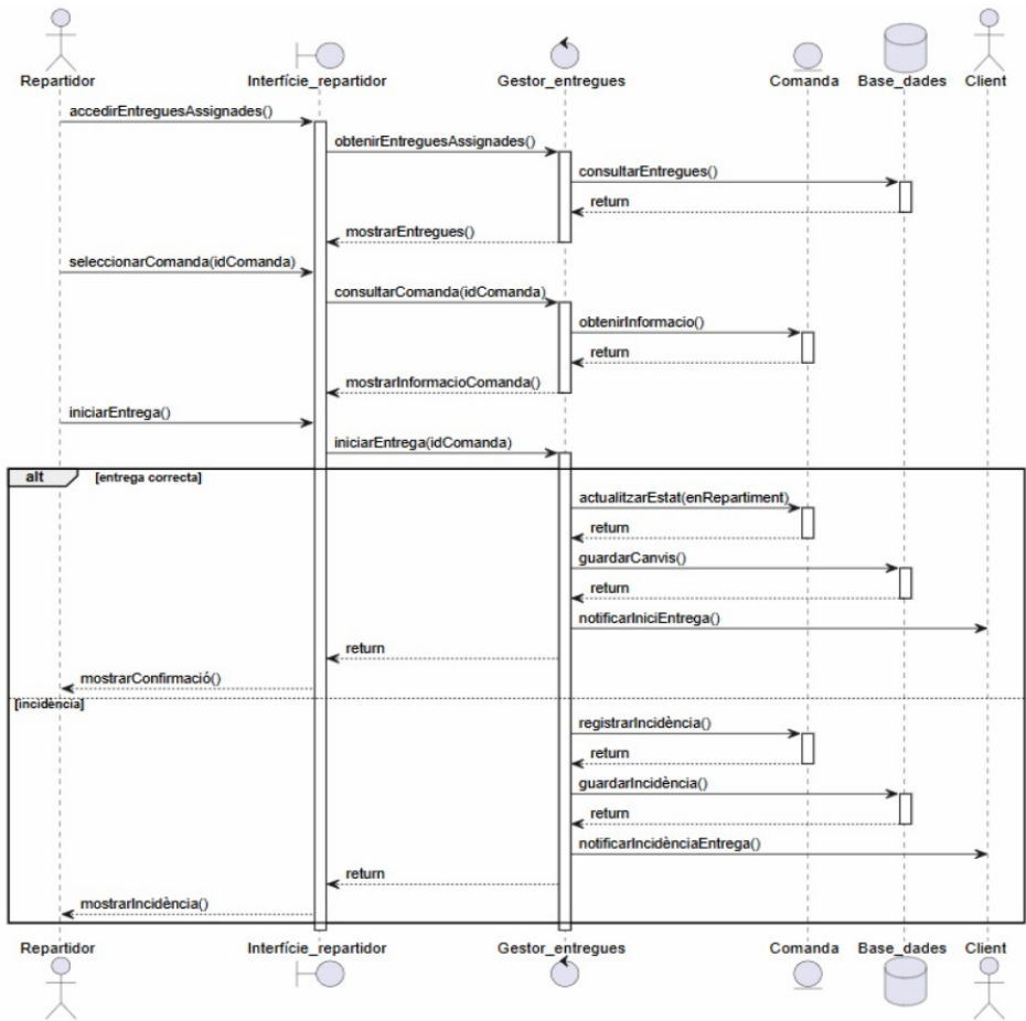
Figura 32. Diagrama de seqüència - Gestionar l'entrega de comandes.
