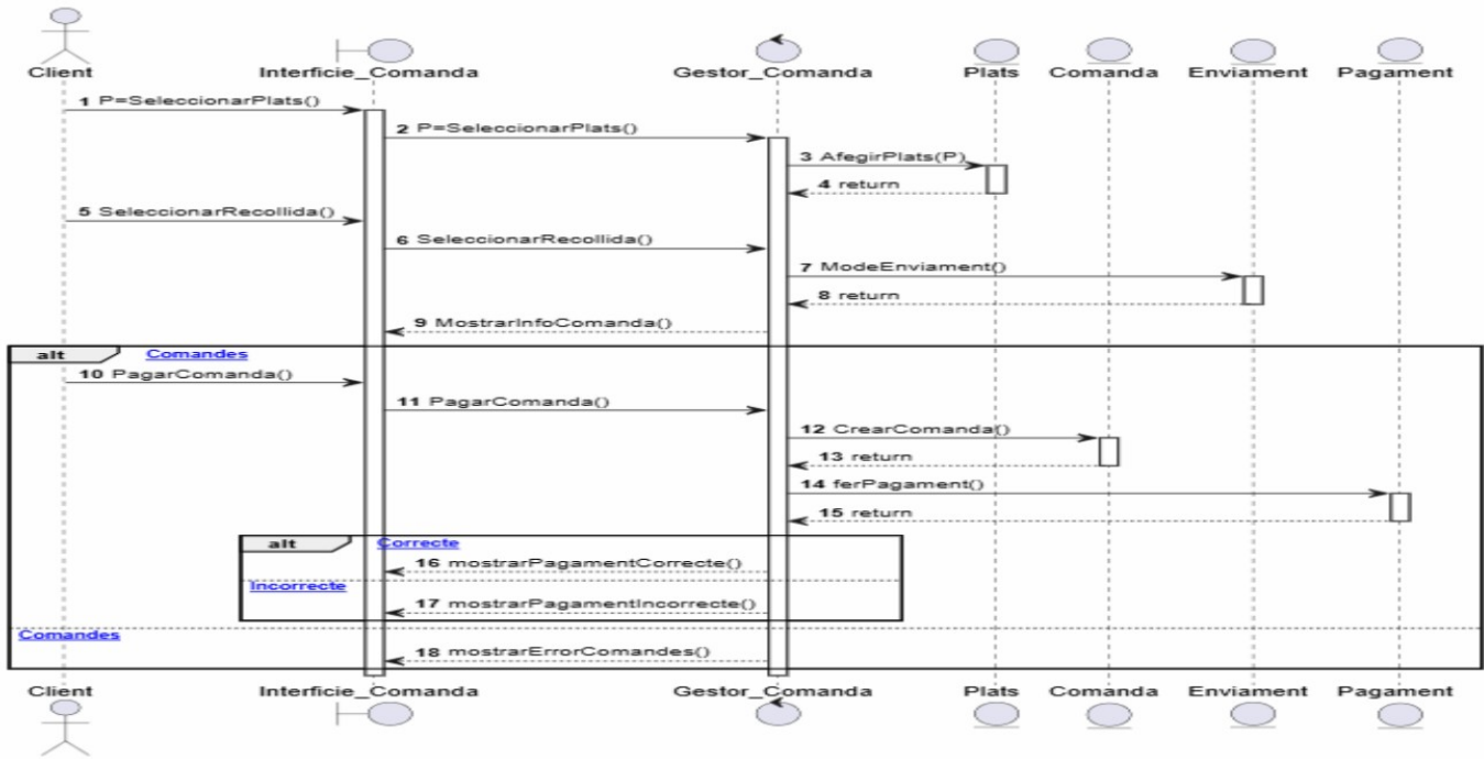
Figura 15. Diagrama de seqüència - Realitzar comanda.
