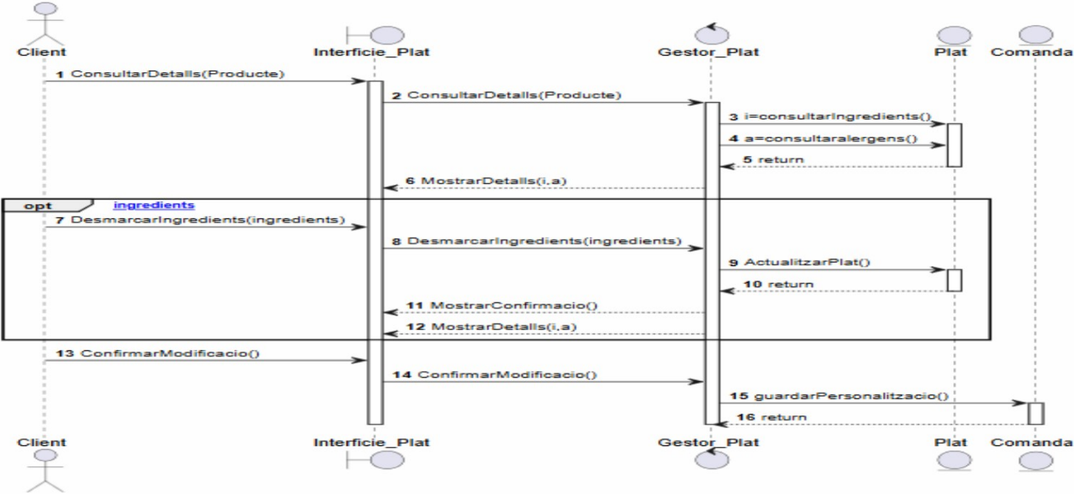
Figura 22. Diagrama de seqüència - Personalitzar plat.
