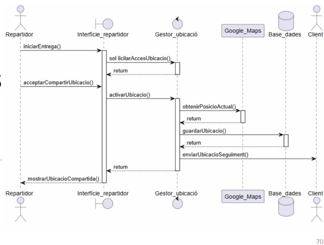
Figura 30. Diagrama de seqüència - Compartir la seva ubicació.
