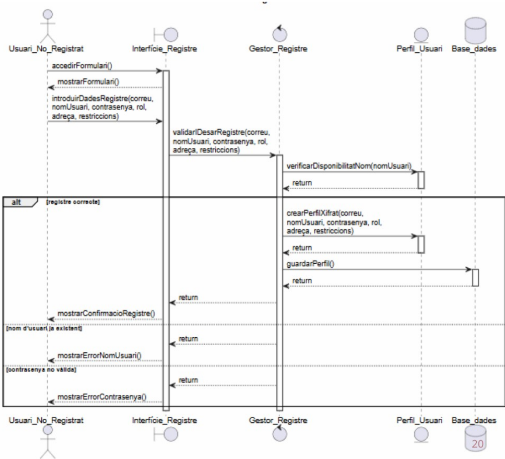
Figura 7. Diagrama de seqüència - Registrar-se.
