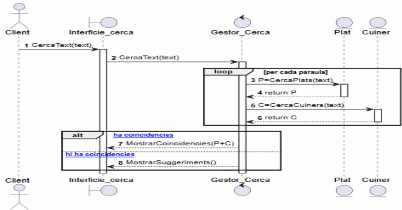
Figura 19. Diagrama de seqüència - Cercar cuiner o plat.
