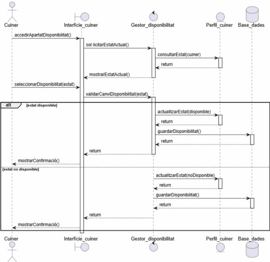
Figura 25. Diagrama de seqüència - Gestionar disponibilitat.
