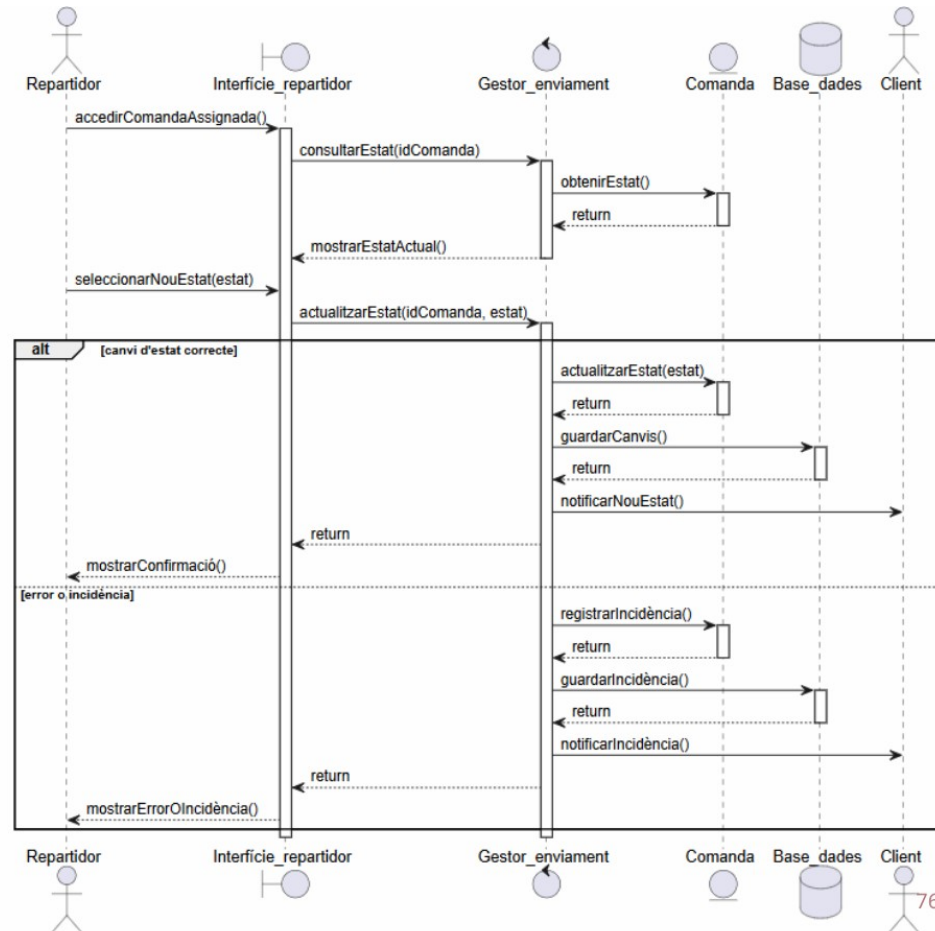
Figura 33. Diagrama de seqüència - Actualitzar l'estat de l'enviament.
