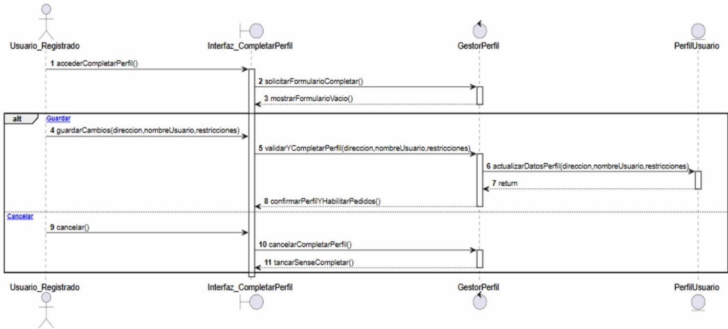
Figura 12. Diagrama de seqüència - Completar Perfil.
