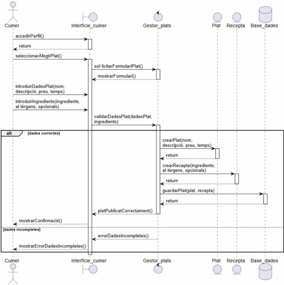
Figura 24. Diagrama de seqüència - Oferir plats i receptes.
