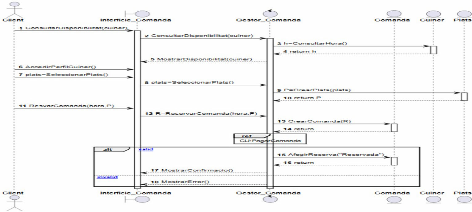
Figura 20. Diagrama de seqüència - Reservar comanda.
