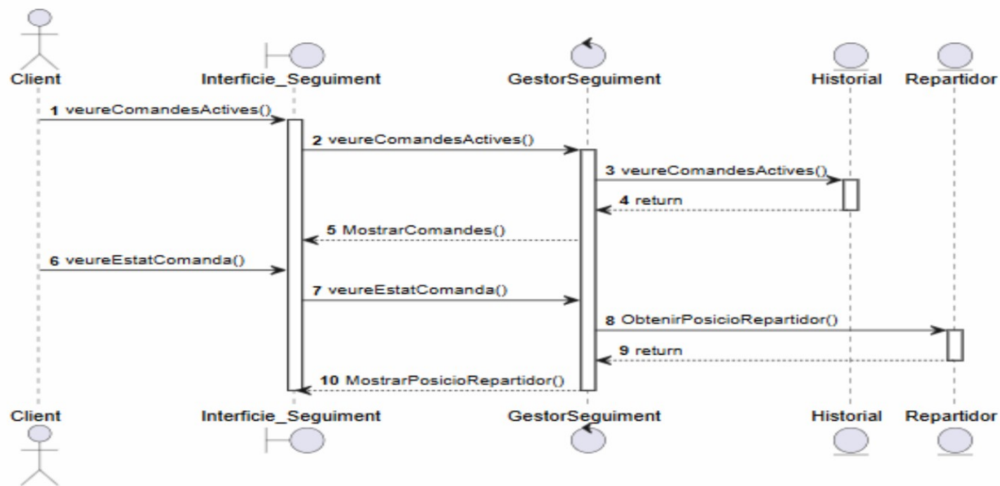
Figura 16. Diagrama de seqüència - Fer seguiment de l'enviament.
