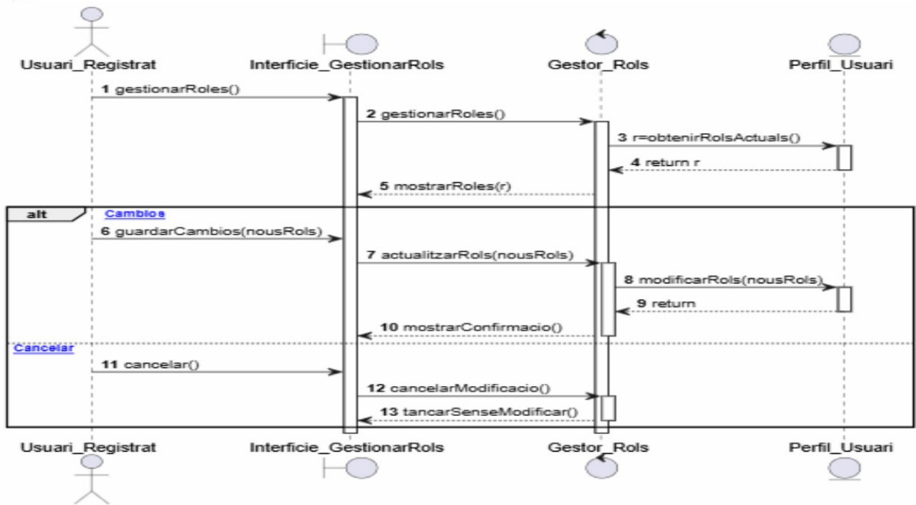
Figura 9. Diagrama de seqüència - Gestionar rols.
