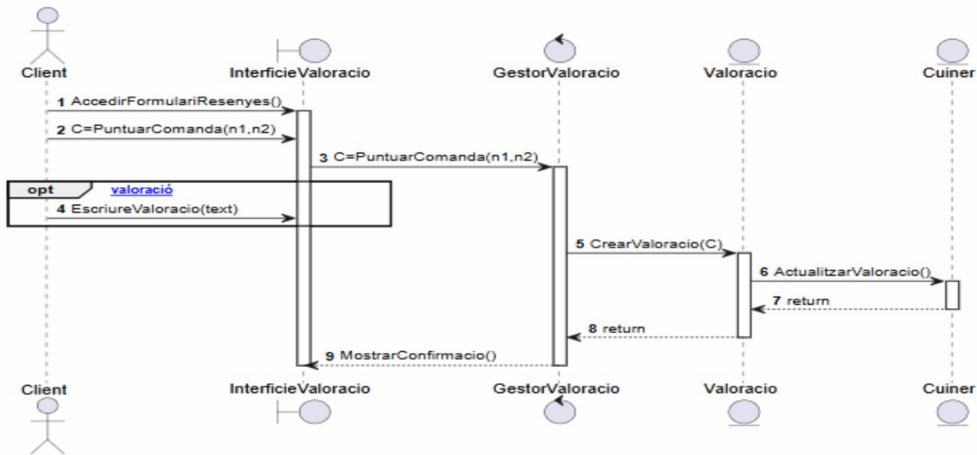
Figura 18. Diagrama de seqüència - Valorar comanda.
