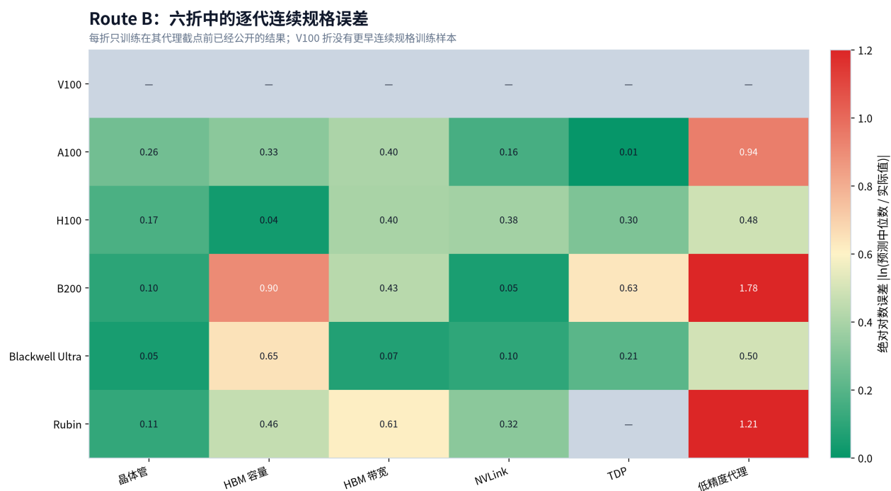
图 13: Route B 严格时点留出折的逐代连续规格绝对对数误差；破折号表示该折无法形成相应连续规格预测。图示结论：晶体管误差在各可评分折相对稳定，低精度代理在 B200 与 Rubin 上明显失配，且并非每个世代都有同样多的训练行。
