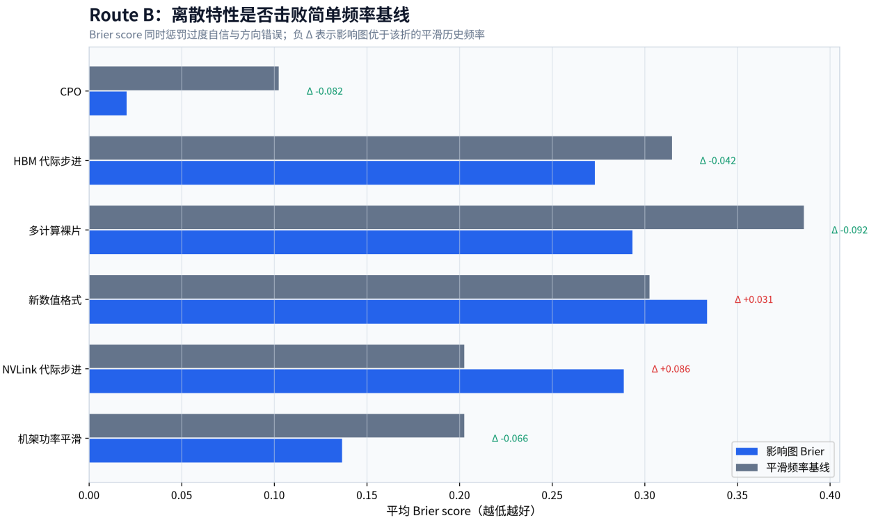
图 15: 六个离散特性节点的平均 Brier score 与同折平滑历史频率基线比较。图示结论：新数值格式与 NVLink 代际步进的 Brier 劣于基线，因此其未来概率不能作为已校准采用率；其余节点的改善也受六折小样本限制。
