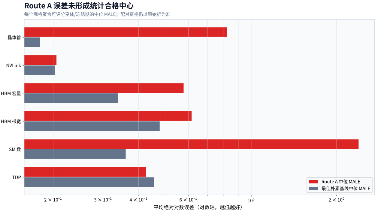
图 10: 可评分规格的 Route A MALE 与同折最佳朴素基线比较；横轴为对数尺度。图示结论：环境代理变量在极小样本上增加方差和外推风险，没有形成优于 last-value 等朴素基线的证据。
