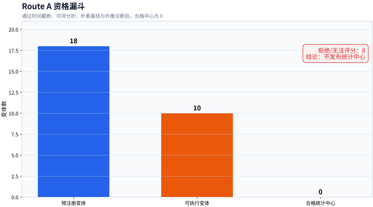
图 9: 18 个预注册变体中 10 个可执行、8 个被拒绝或无可评分析，0 个满足统计中心发布门槛。图示结论：历史样本没有支持可发布的统计预测中心；这一负结果优先于任何漂亮的外推数值。
