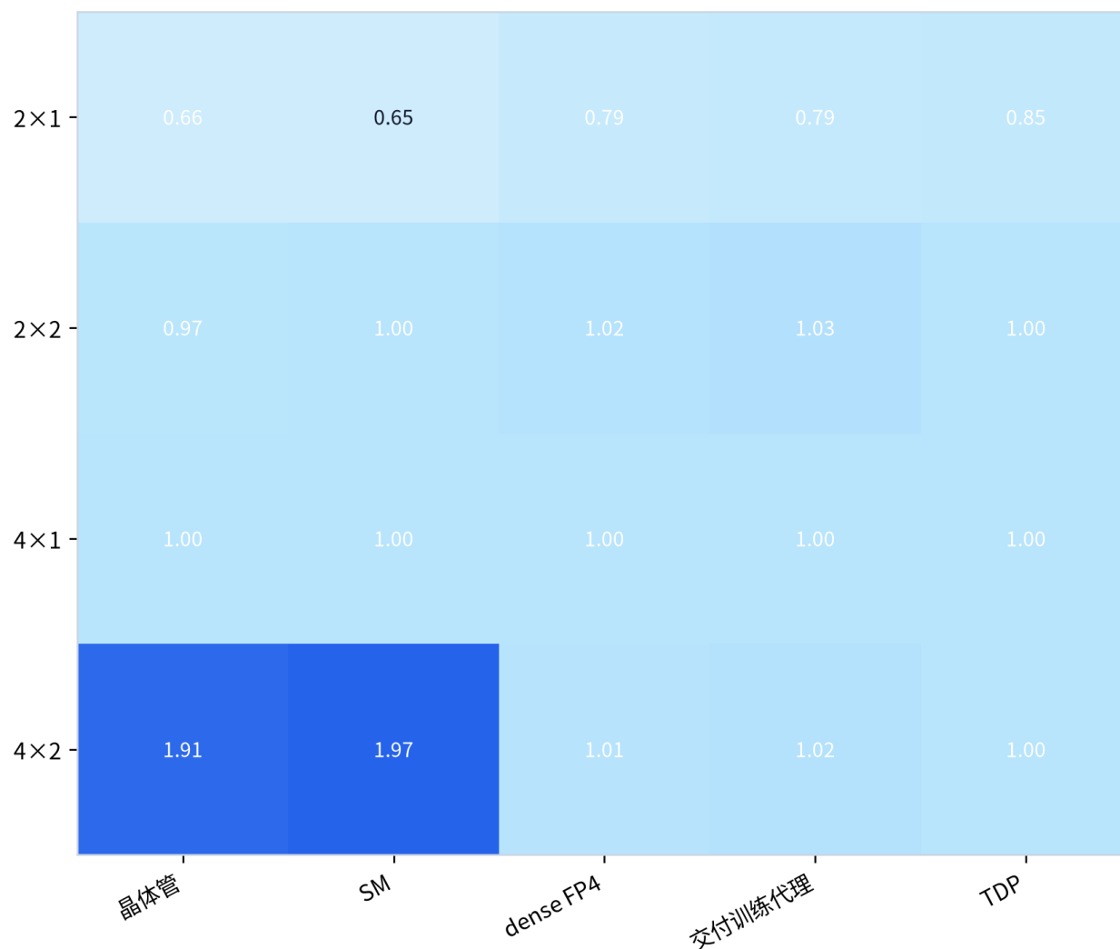
图 22: 四种固定架构在 24 个月 balanced 条件下相对 4\times 1 情景的 q50 比值。图示结论: 4\times 2 将晶体管与 SM 近乎翻倍, 却没有带来同量级 dense FP4 或交付训练增益; 这是模型内的设计压力上界, 不是产品预测。
