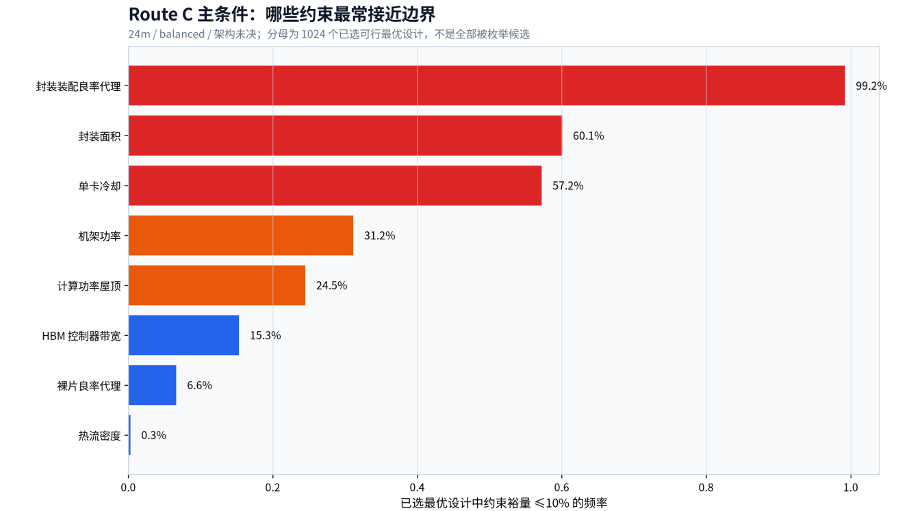
图 19: 24 个月 balanced/架构未决条件下，已选最优设计的约束裕量不超过 10% 的频率。图示结论：封装装配良率代理在 99.2% 的已选设计上接近边界，封装面积与单卡冷却分别约为 60.1% 和 57.2%，构成主工作点的主要工程依赖。
