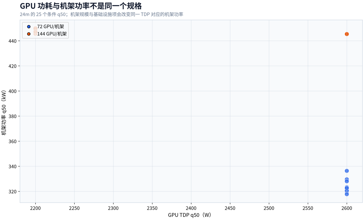
图 23: 24 个月 25 个工程条件的 GPU TDP q50 与机架功率 q50，颜色区分 72/144 GPU 机架。图示结论：把单 GPU TDP 直接乘 GPU 数会遗漏基础设施、利用率和电源转换条件；机架层预测必须单列。
