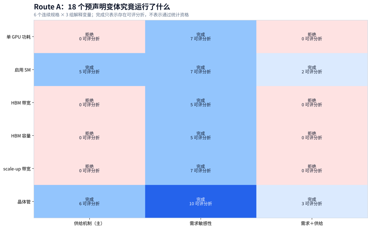
图 6: Route A 的六个规格与三种预声明解释变量组合；单元格给出可评分历史折数，红色表示所有候选折均无法构造。图示结论：10 个变体完成数值拟合、8 个变体在拟合前因无可评分析被拒绝；完成不等于获得预测中心资格。
