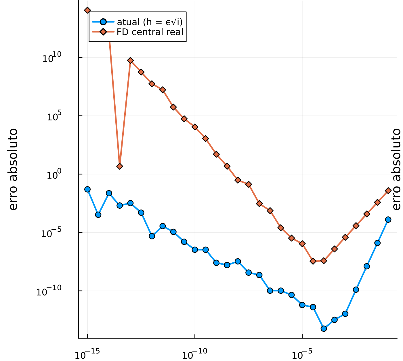
2ª derivada \partial^2 f/\partial x^2 — erro vs passo
