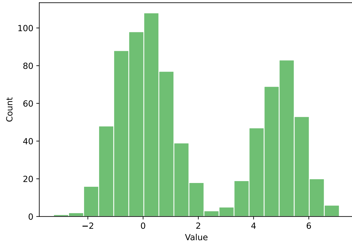
ATCND optimal: 19 bins
