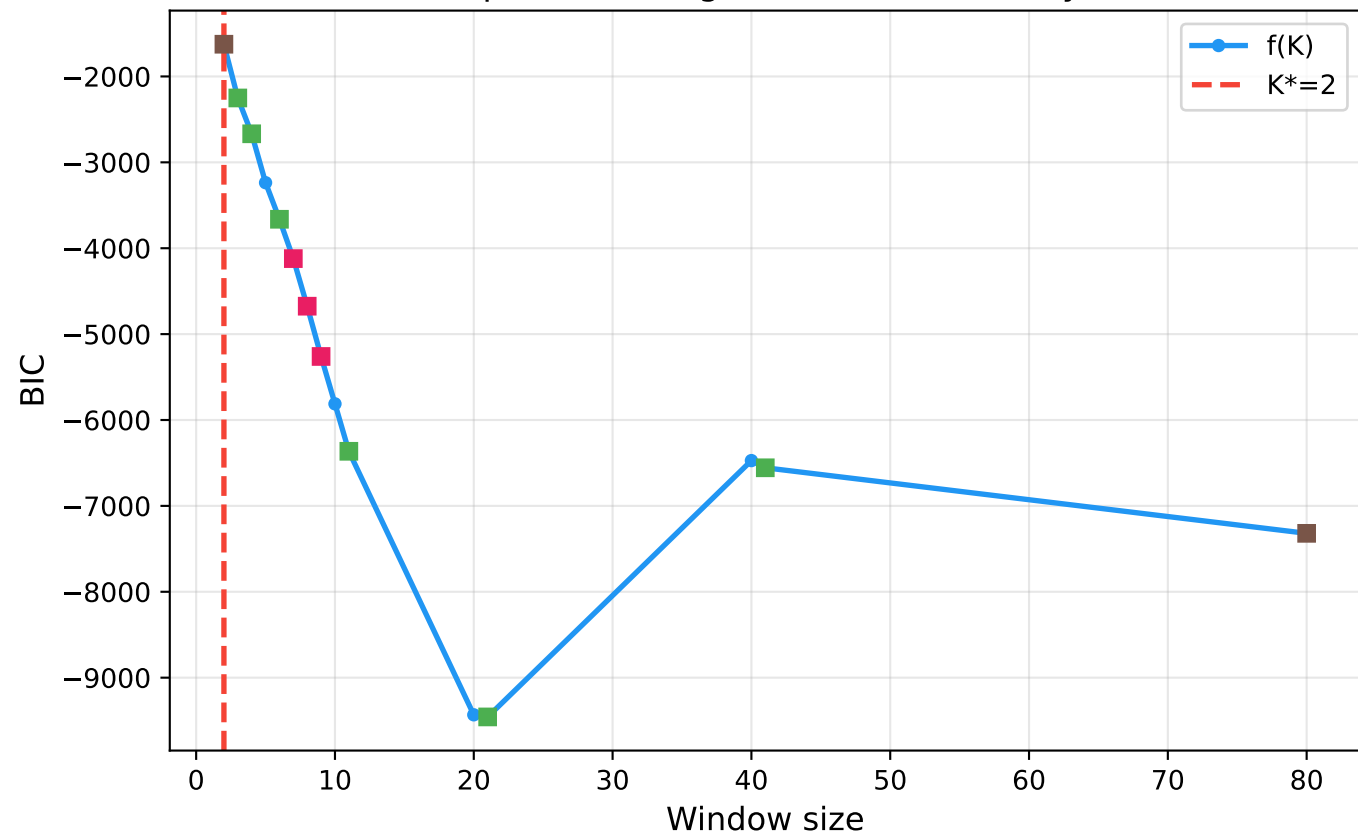
Pandas: Optimal Rolling Window (BIC, binary search)
