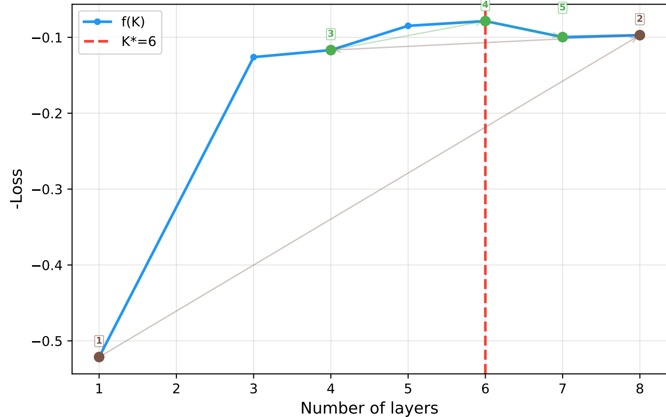
PyTorch: Hidden Layer Count (-CE loss)
