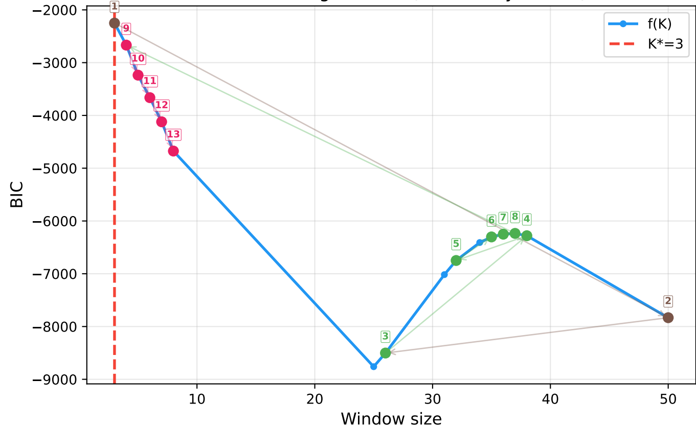
Pandas: Rolling Window (BIC, binary search)
