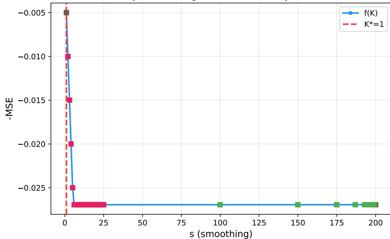
SciPy: Smoothing Parameter (binary search)
