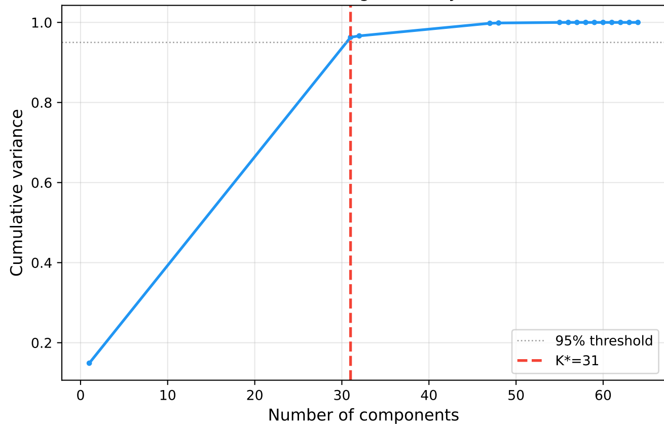
sklearn: PCA on Digits (binary search)
