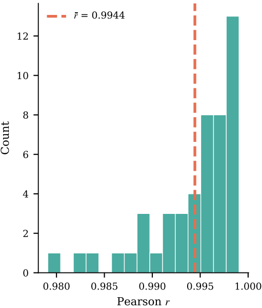
(c) Cross-Axis r (Lang \times Disc)
