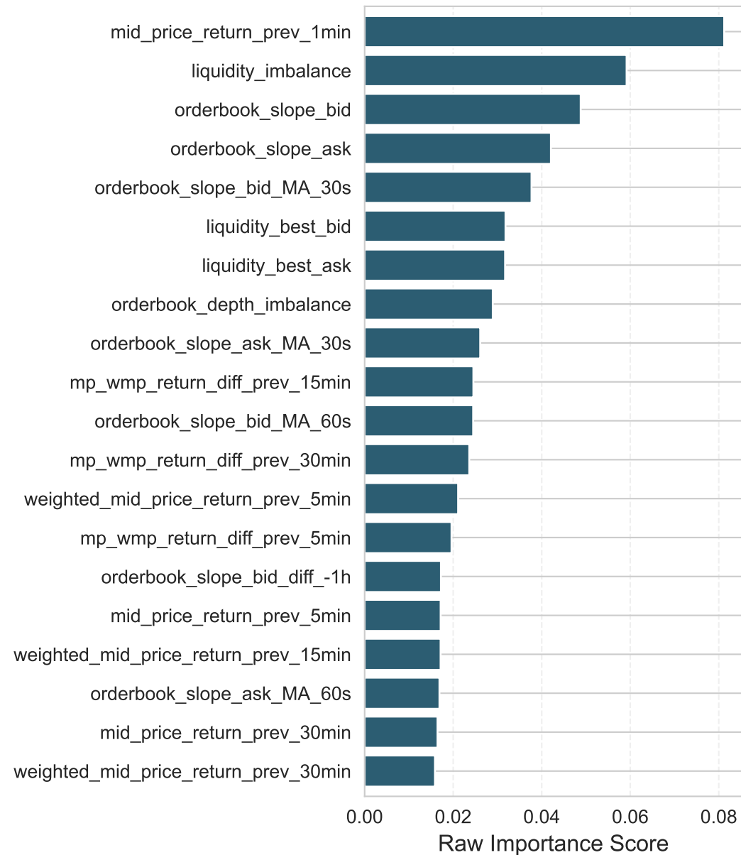
Random Forest (Gini Importance / Raw)
