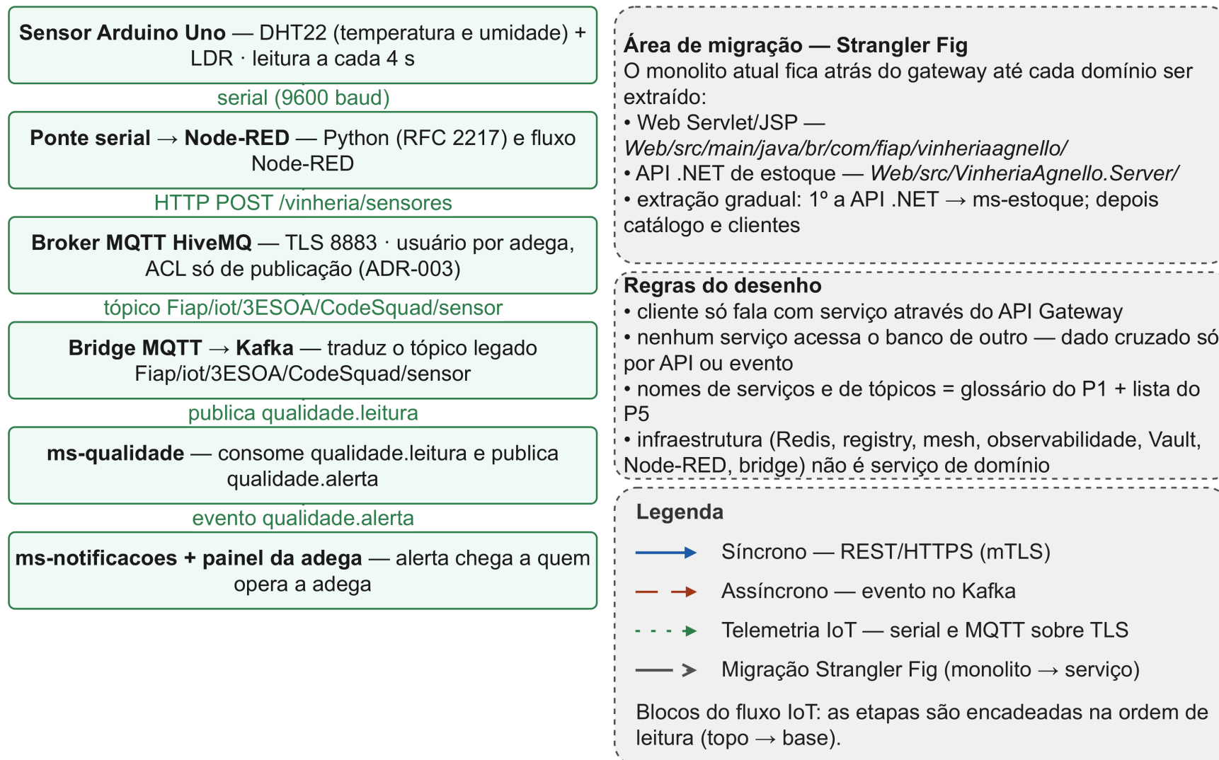
Figura 4 — Detalhe 3: fluxo IoT da adega (sensor → MQTT → bridge → Kafka) e migração do monolito
