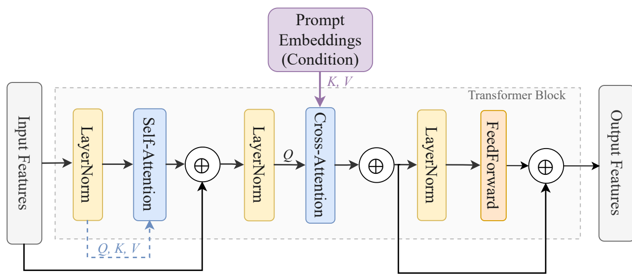
(d) Basic TransformerBlock w/ SA
