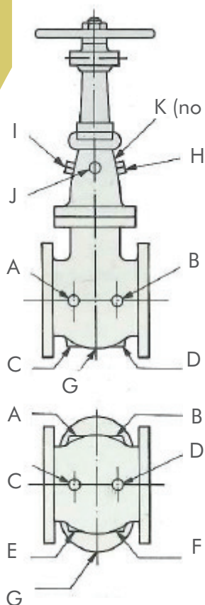
VÁLVULA GAVETA
