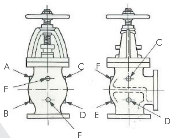
VÁLVULA ANGULAR
