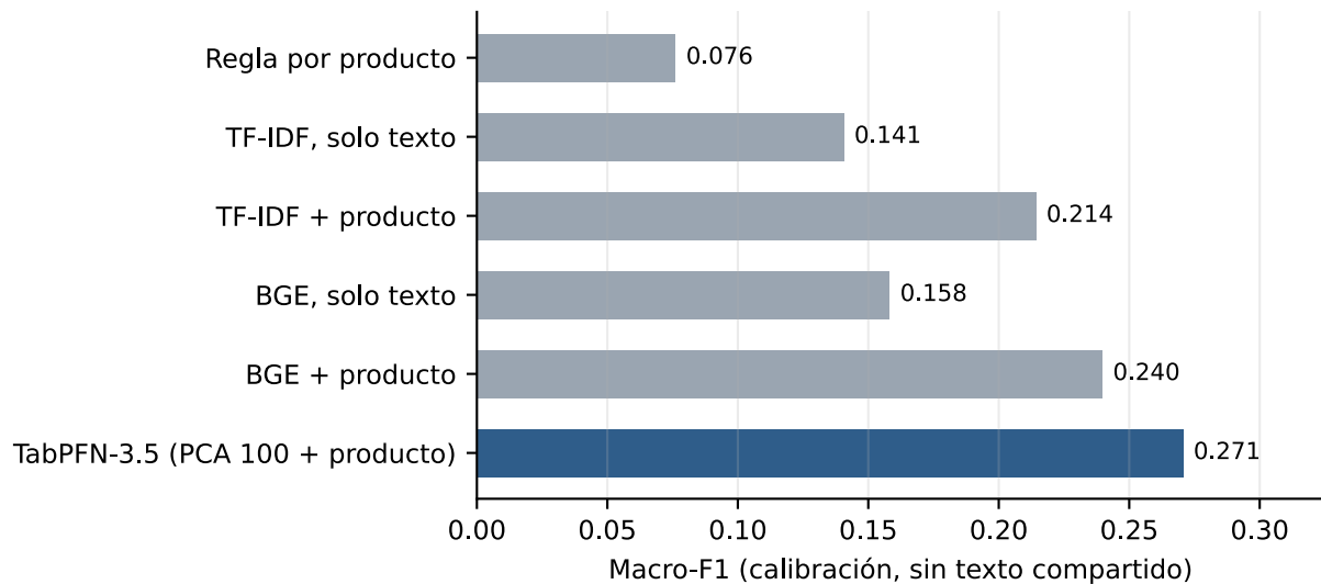
Figura 2: Macro-F1 de T1 en calibración por representación. El producto y los embeddings aportan; TabPFN-3.5 sobre PCA 100 más producto es el vigente.
