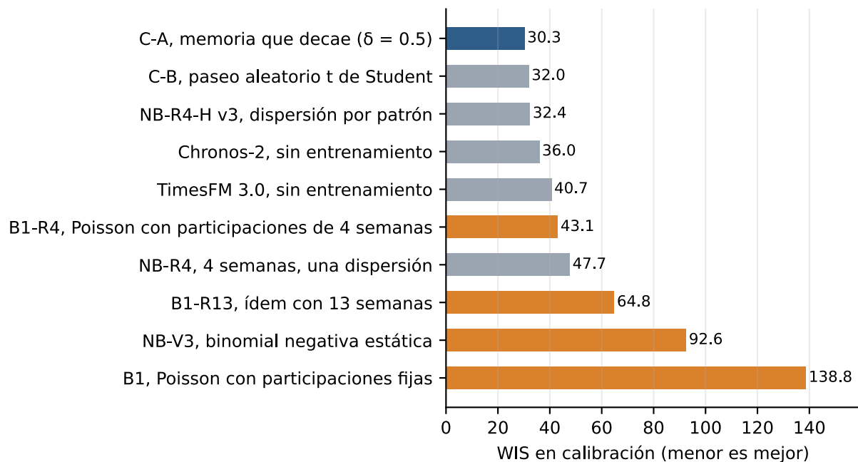
Figura 7: WIS de calibración de los candidatos semanales. C-A, la binomial negativa jerárquica con memoria que decae, es la vigente.
