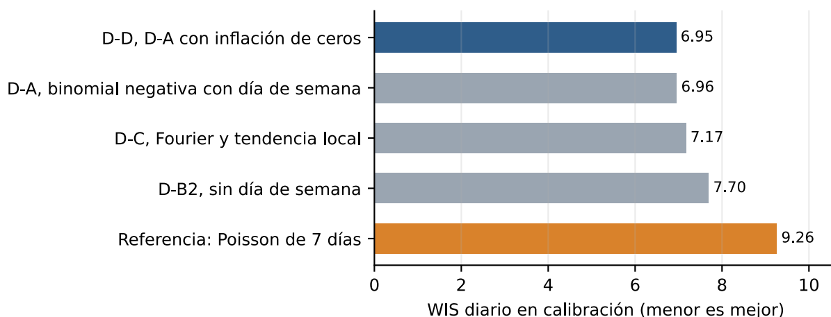
Figura 10: WIS diario de calibración de los candidatos de conteo y de la referencia Poisson de 7 días.
