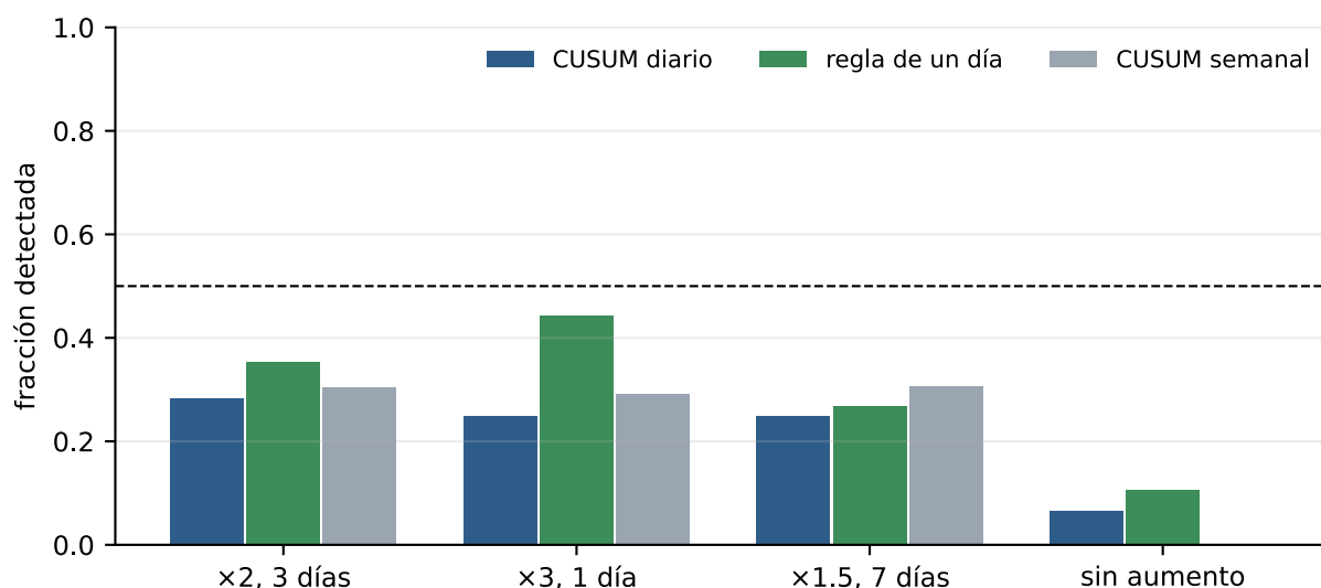
Figura 11: Fracción de ráfagas detectadas por cada regla diaria y por el CUSUM semanal. Ninguna regla diaria alcanza el 50 % exigido.
