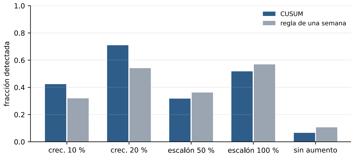
Figura 9: Fracción detectada por escenario y regla. CUSUM gana en los dos crecimientos sostenidos, que son los que deciden.
