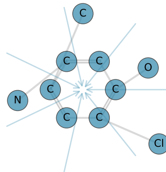
c Set2Set
