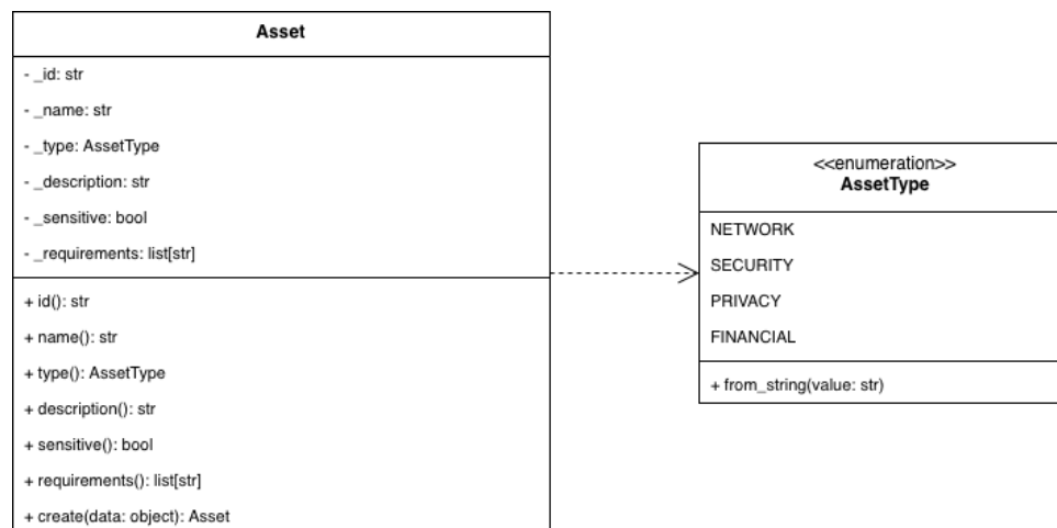
Figura 32: Asset G : classe backend G
