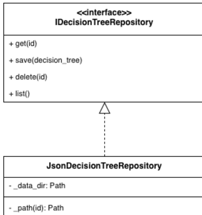
Figura 25: JsonDecisionTreeRepository: classe persistence
