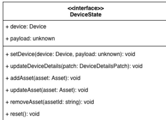
Figura 15: DeviceStore: Store state management
