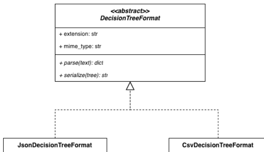
Figura 20: decision_tree_format: interfaccia G e realizzazioni
