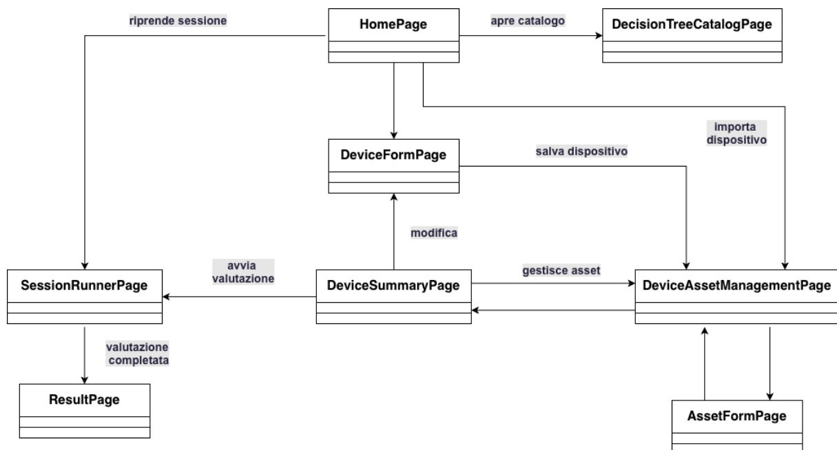
Figura 2: Diagramma delle pagine
