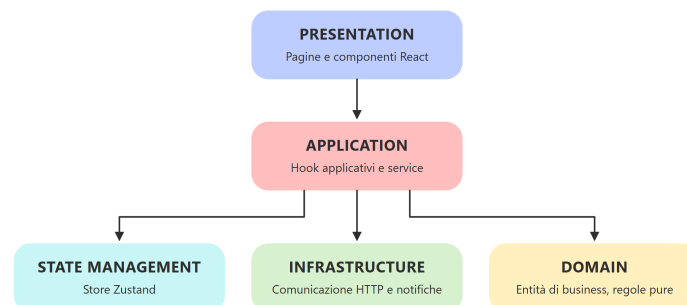
Figura 1: Diagramma a blocchi dei livelli del frontend G
