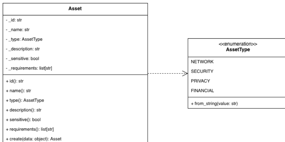
Figura 29: Asset_G : classe backend
