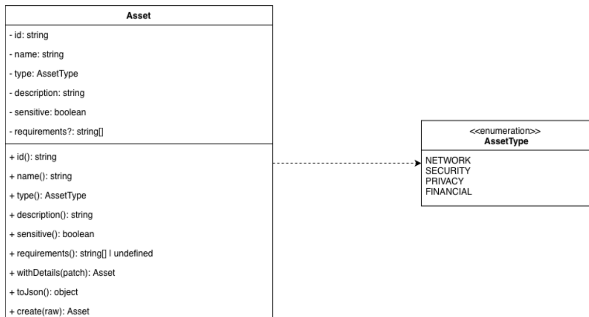
Figura 24: Asset G : classe frontend G
