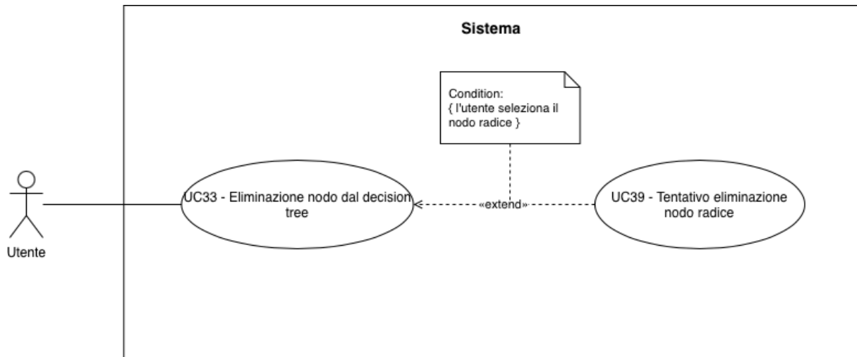
UC-33 : Eliminazione nodo G dal decision tree G
