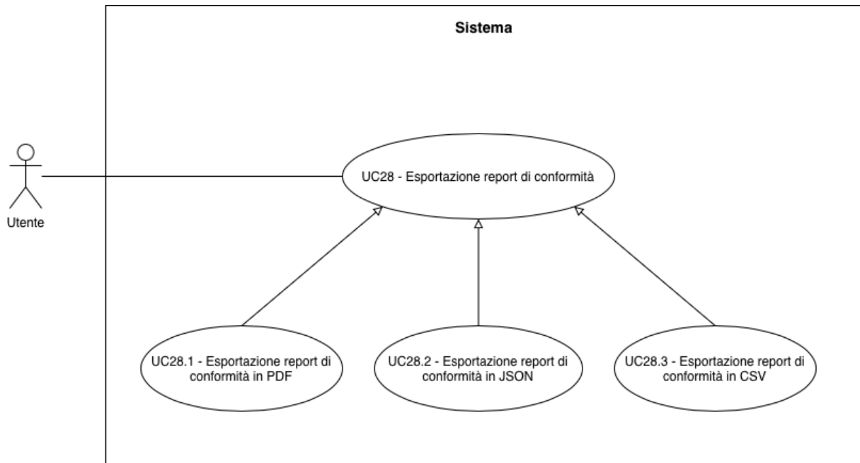
UC-28 : Esportazione G report di conformità G
