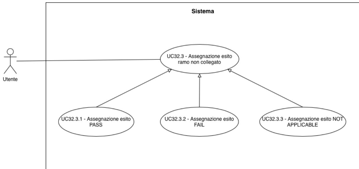
UC-32.3 : Assegnazione esito ramo non collegato
