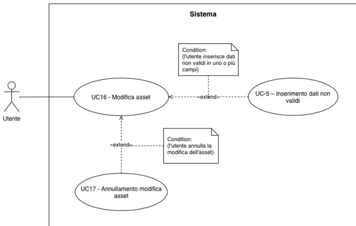
UC-16 : Modifica asset G
