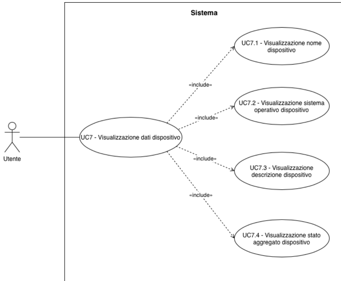
UC-7 : Visualizzazione dati dispositivo
