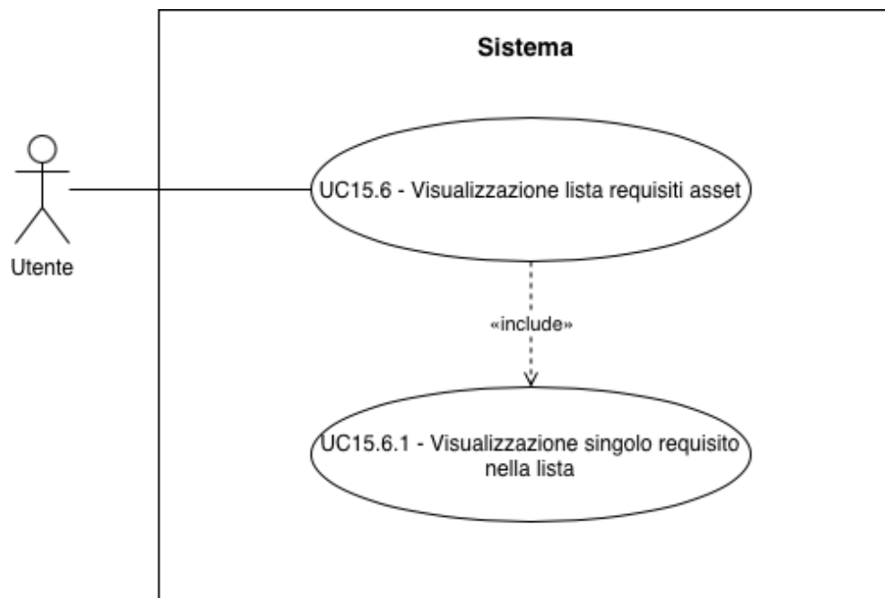
UC-15.6 : Visualizzazione lista requisiti G asset G
