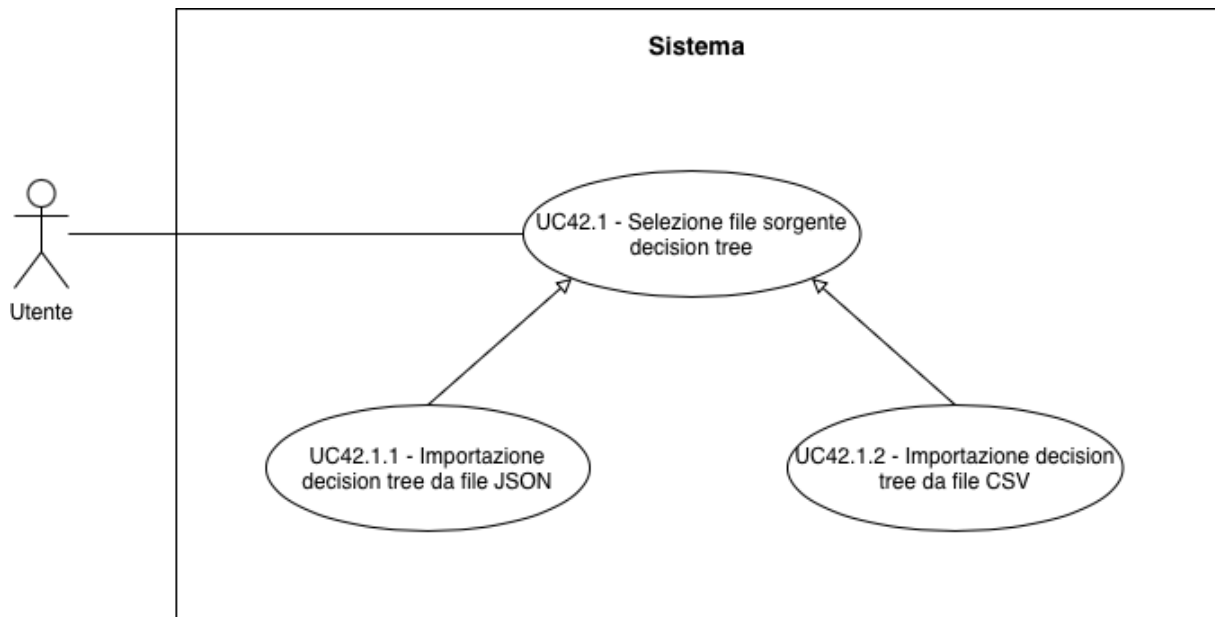
UC-42.1 : Selezione file sorgente decision tree G
