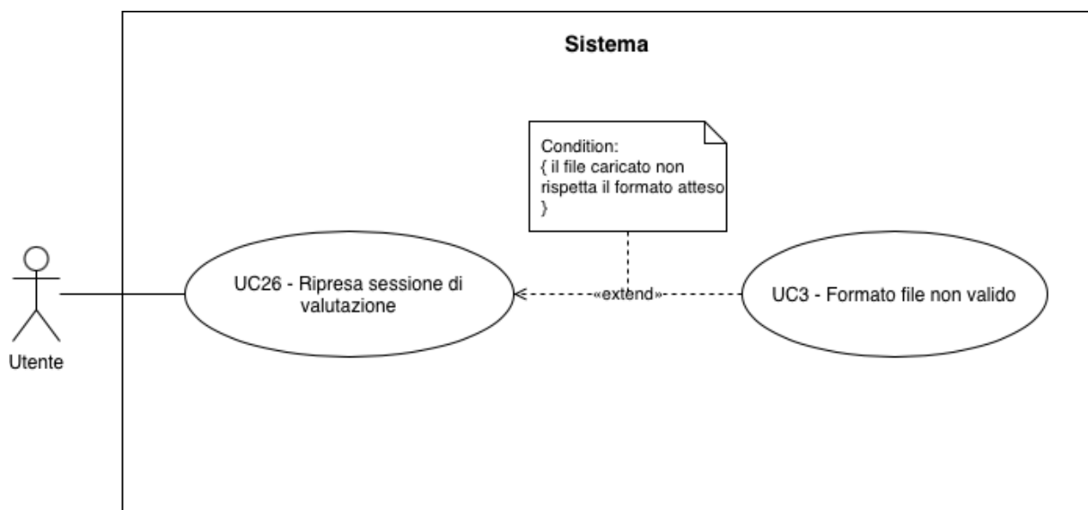
UC-26 : Ripresa sessione di valutazione G
