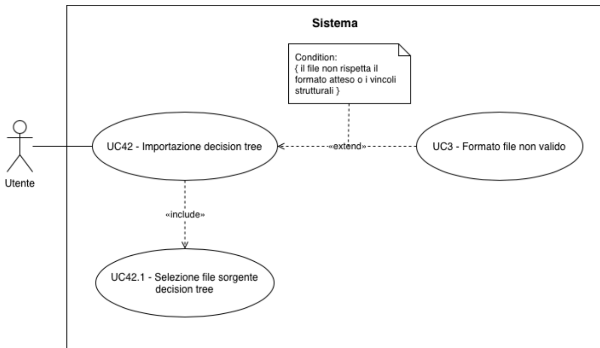
UC-42 : Importazione G decision tree G
