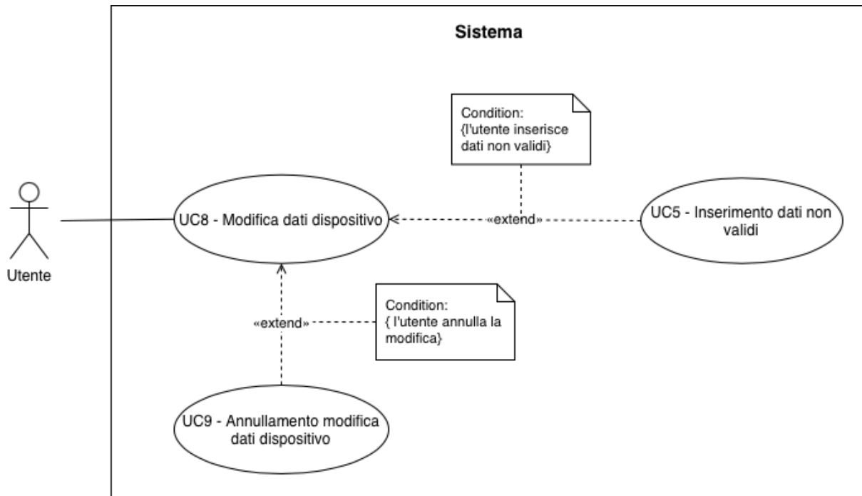
UC-8 : Modifica dati del dispositivo
