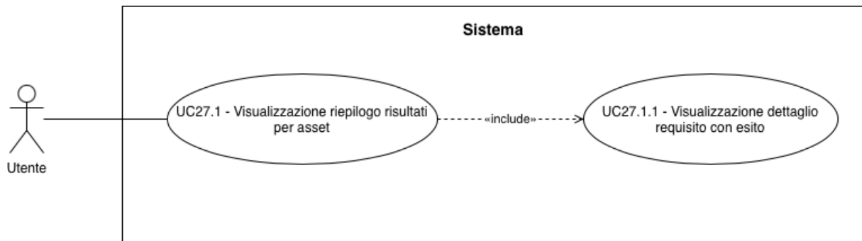
UC-27.1 : Visualizzazione riepilogo risultati per asset
