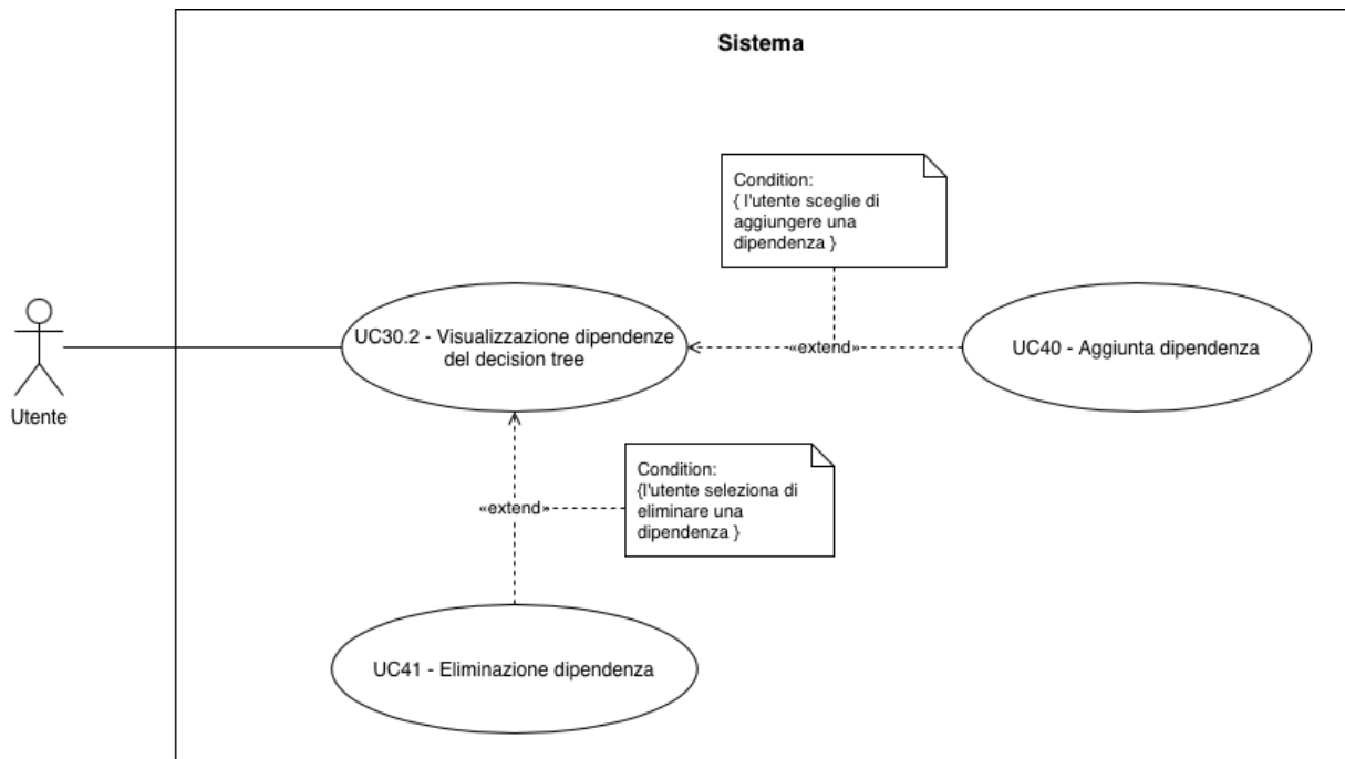
UC-30.2 : Visualizzazione dipendenze del decision tree G
