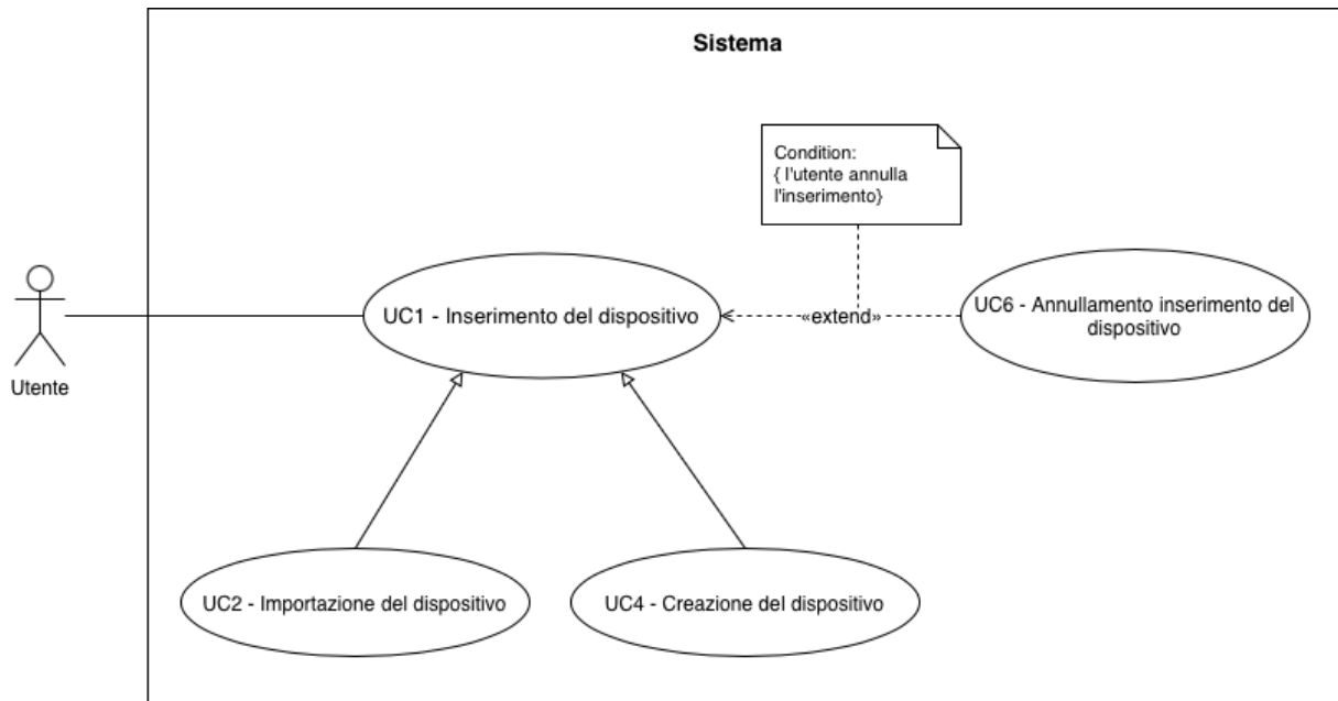
UC-1 : Inserimento del dispositivo
