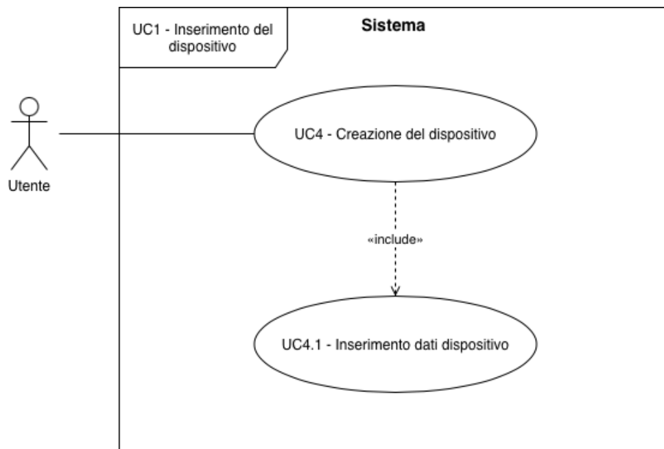
UC-4 : Creazione del dispositivo
