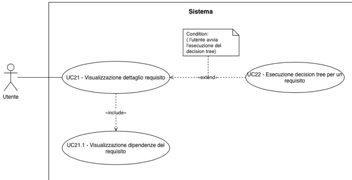
UC-21 : Visualizzazione dettaglio requisito
