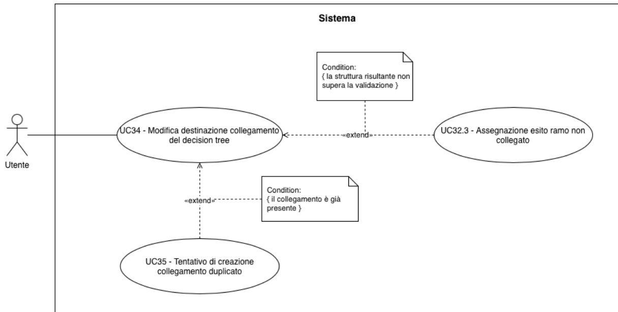
UC-34 : Modifica destinazione collegamento del decision tree G
