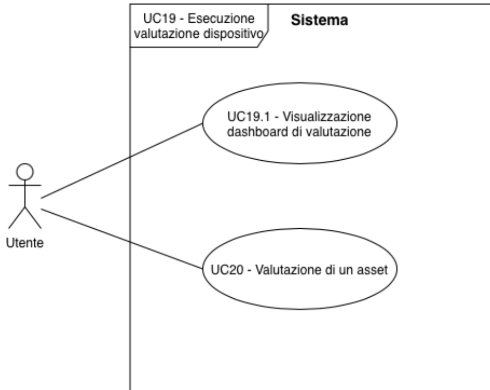
UC-19.1 : Dashboard G e valutazione asset G
