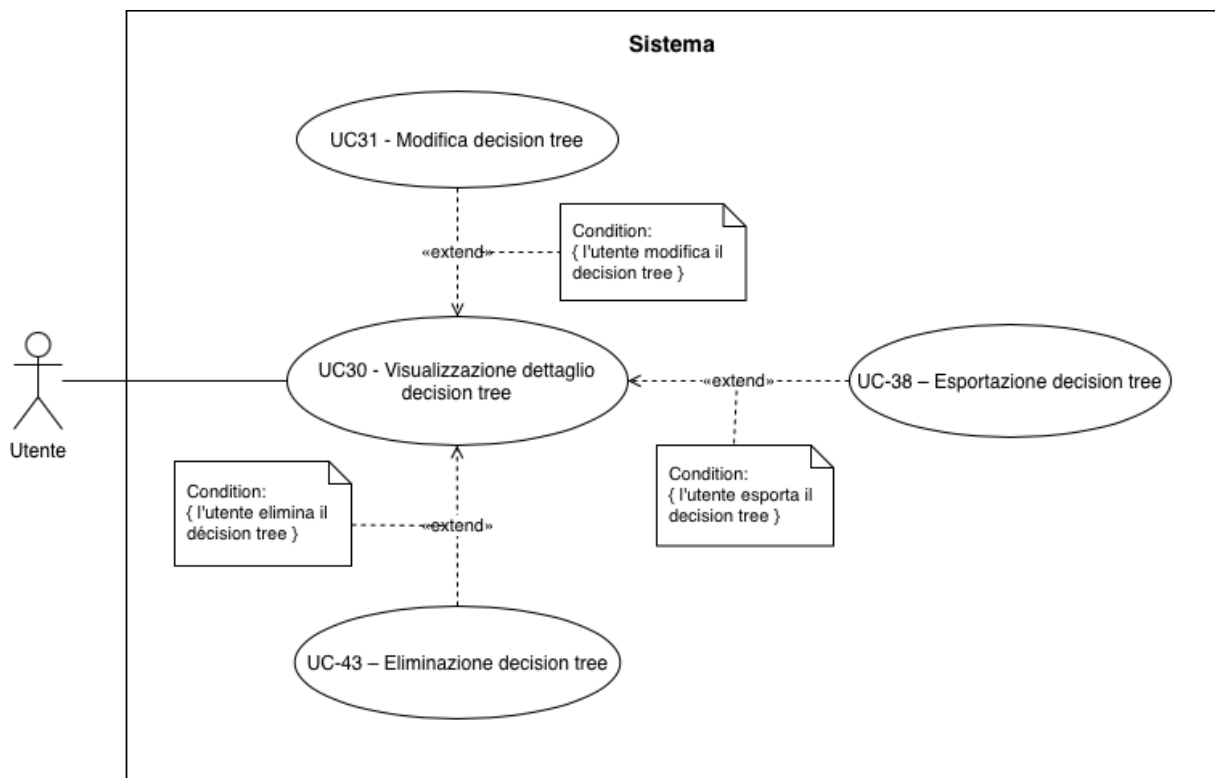
UC-30 : Visualizzazione dettaglio del decision tree G
