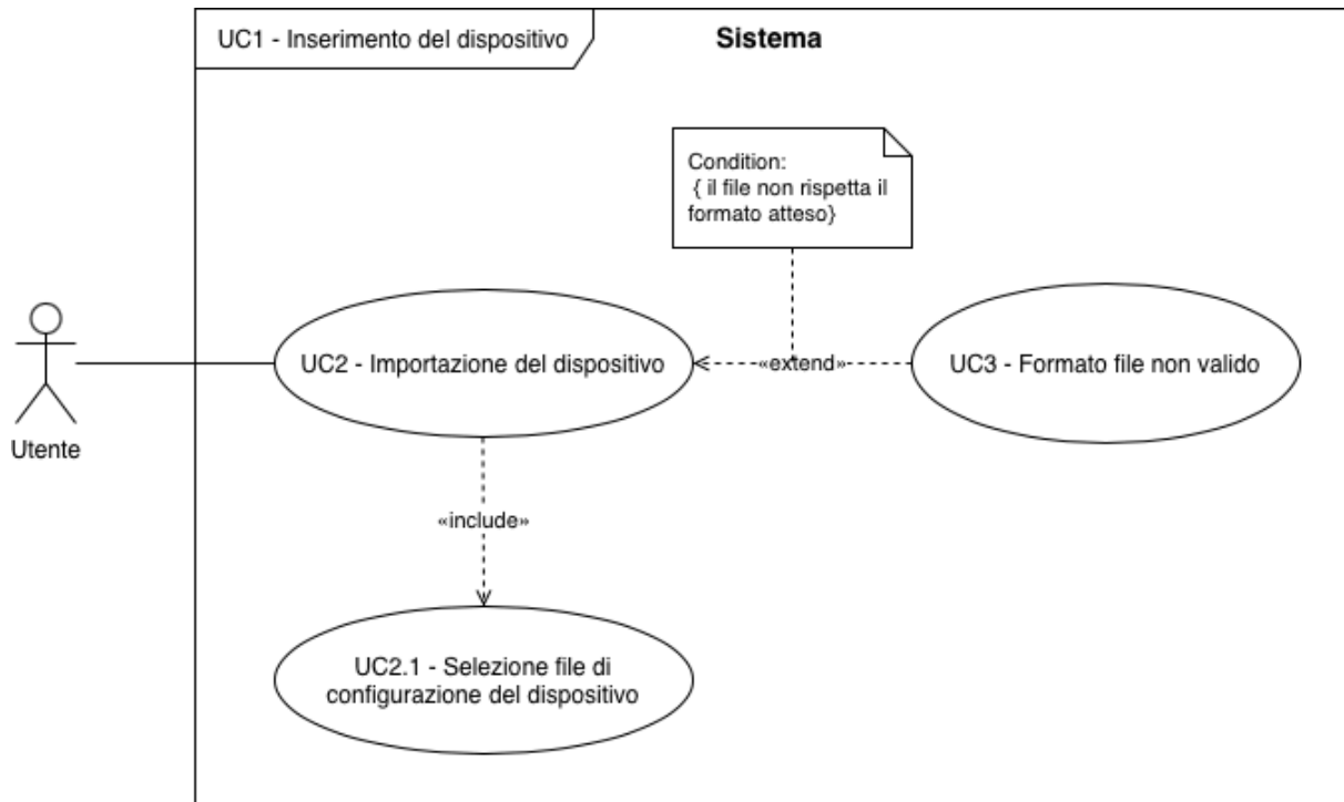
UC-2 : Importazione G del dispositivo
