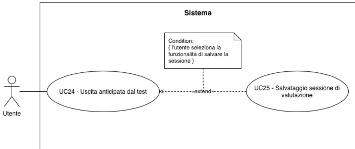
UC-24 : Uscita anticipata dal test
