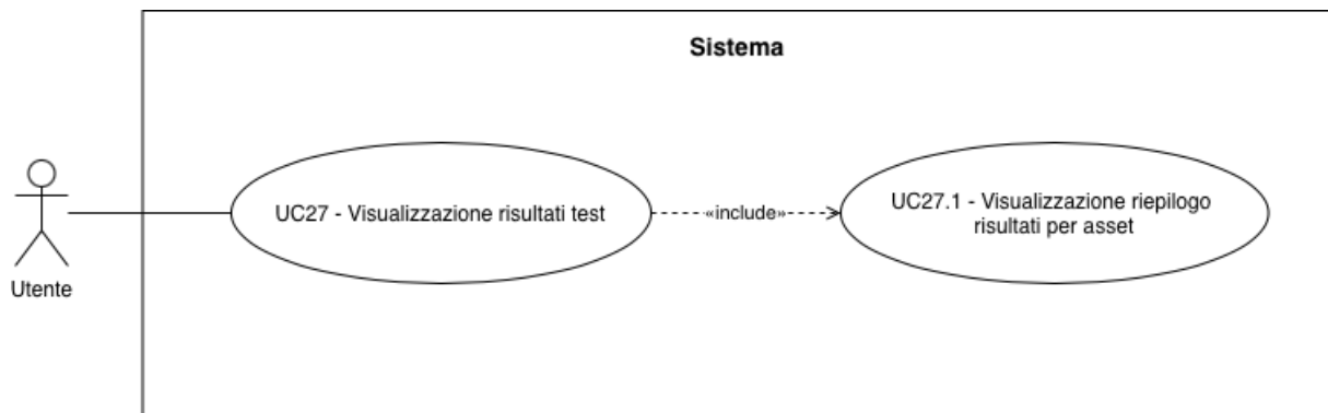
UC-27 : Visualizzazione risultati test
