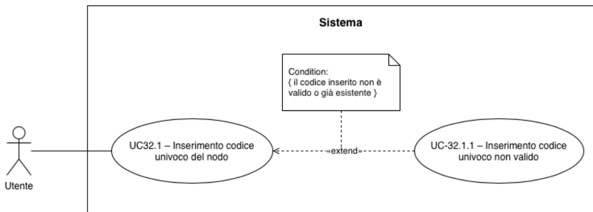
UC-32.1 : Inserimento codice univoco del nodo
