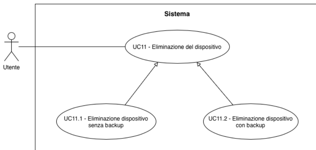
UC-11 : Eliminazione del dispositivo
