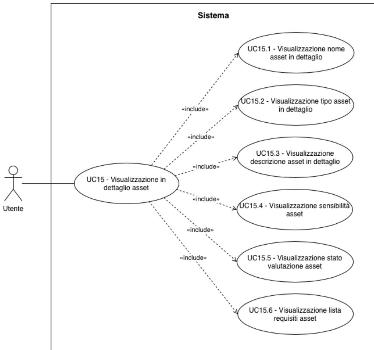
UC-15 : Visualizzazione in dettaglio asset G
