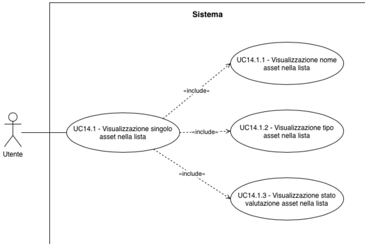
UC-14.1 : Visualizzazione singolo asset G nella lista
