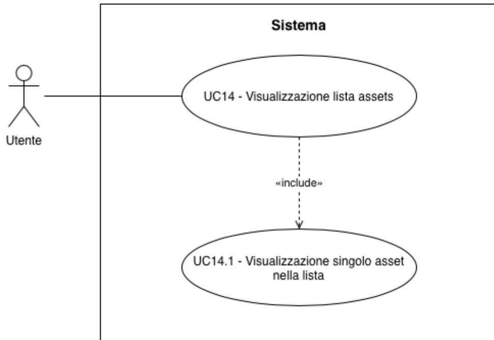
UC-14 : Visualizzazione lista asset G
