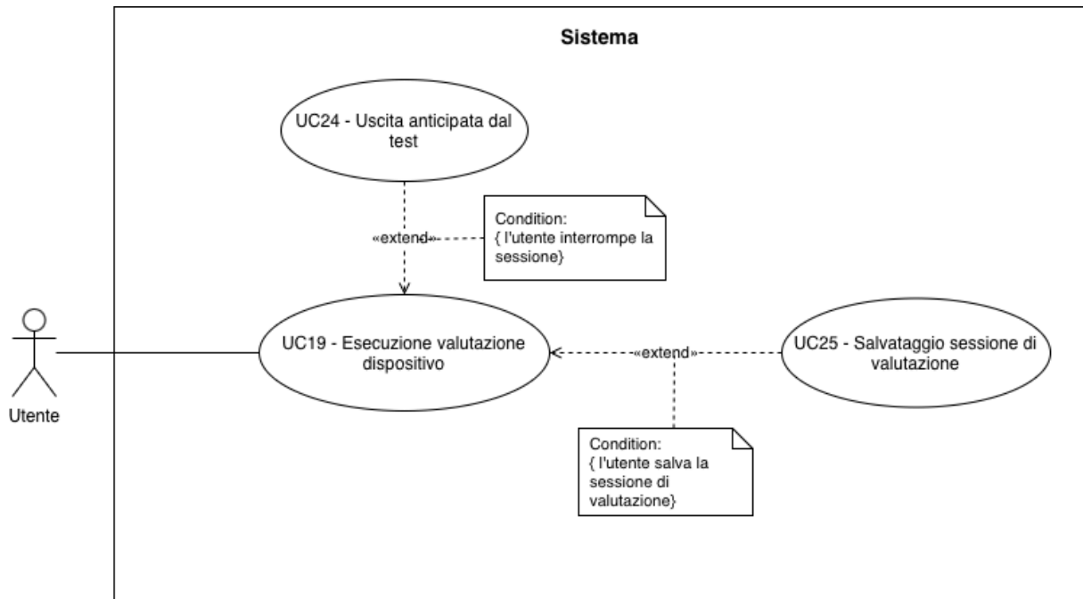
UC-19 : Esecuzione valutazione dispositivo
