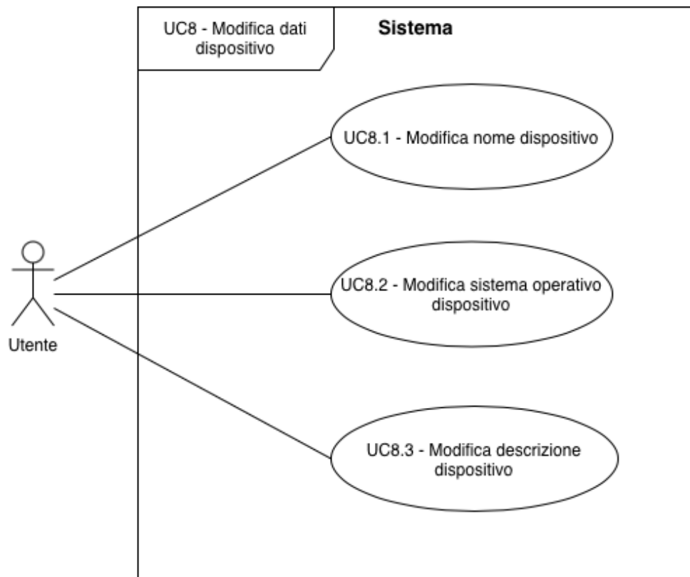
UC-8 : Modifica nome, SO e descrizione del dispositivo
