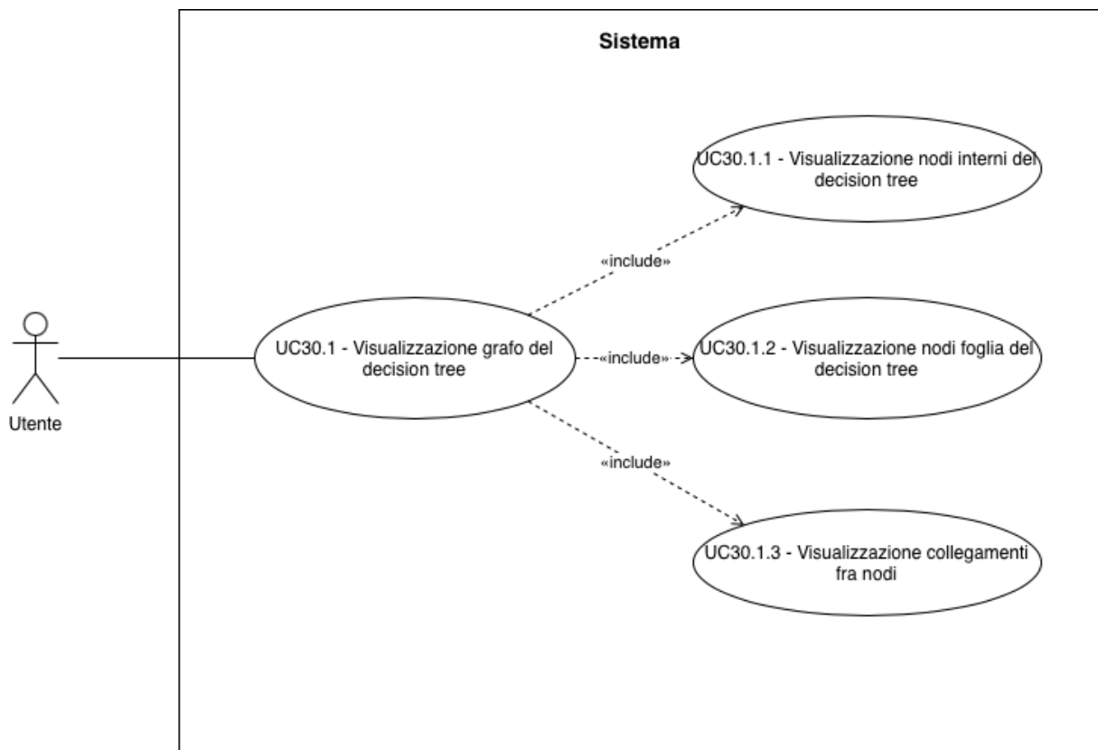
UC-30.1 : Visualizzazione grafo G del decision tree G
