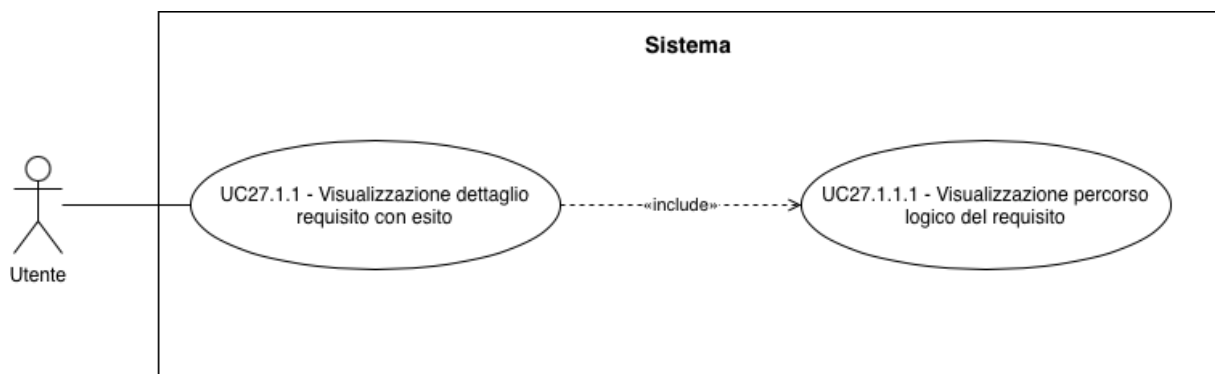
UC-27.1.1 : Visualizzazione singolo requisito con esito
