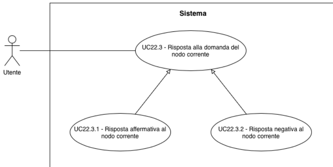
UC-22.3 : Risposta alla domanda del nodo G corrente
