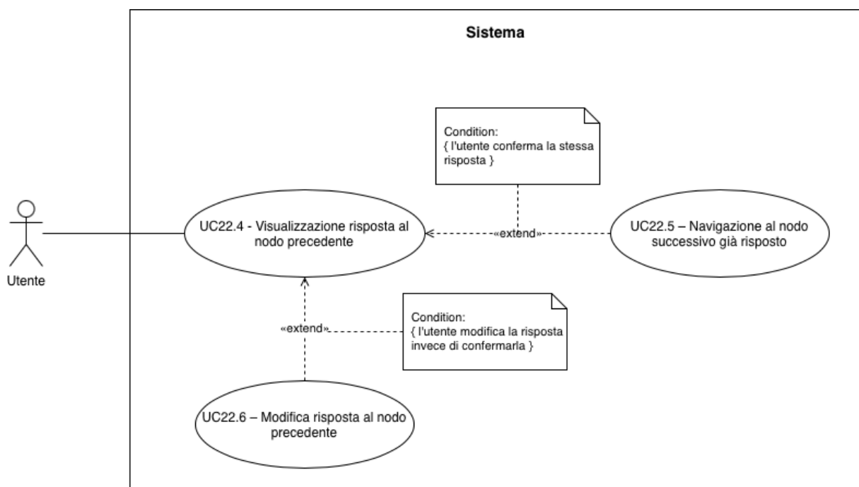
UC-22.4 : Visualizzazione risposta al nodo G precedente
