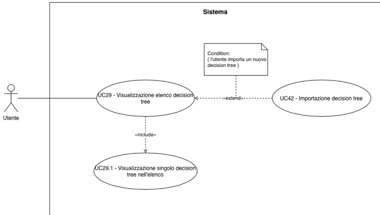
UC-29 : Visualizzazione elenco decision tree G
