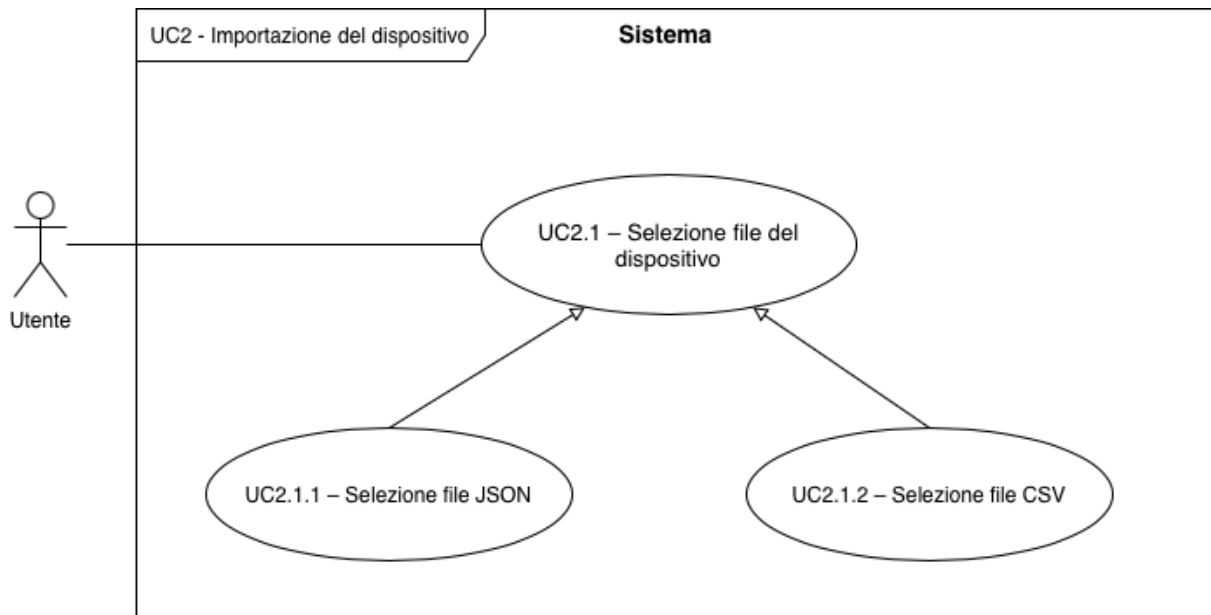
UC-2.1 : Selezione file del dispositivo
