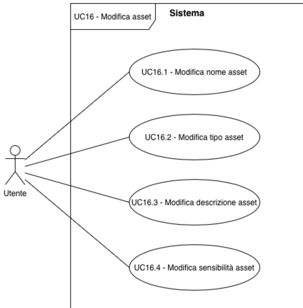
UC-16 : Modifica nome, tipo, descrizione e sensibilità G asset G
