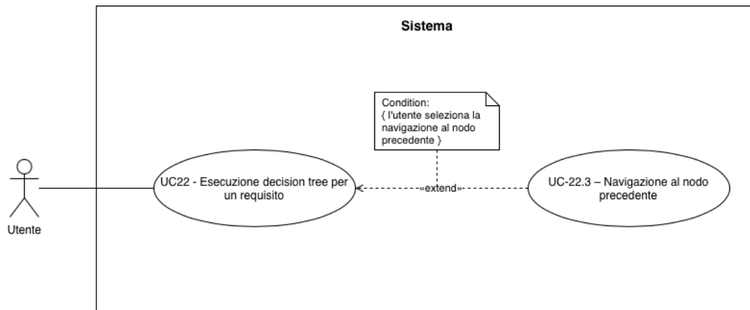
UC-22 : Esecuzione decision tree G per un requisito
