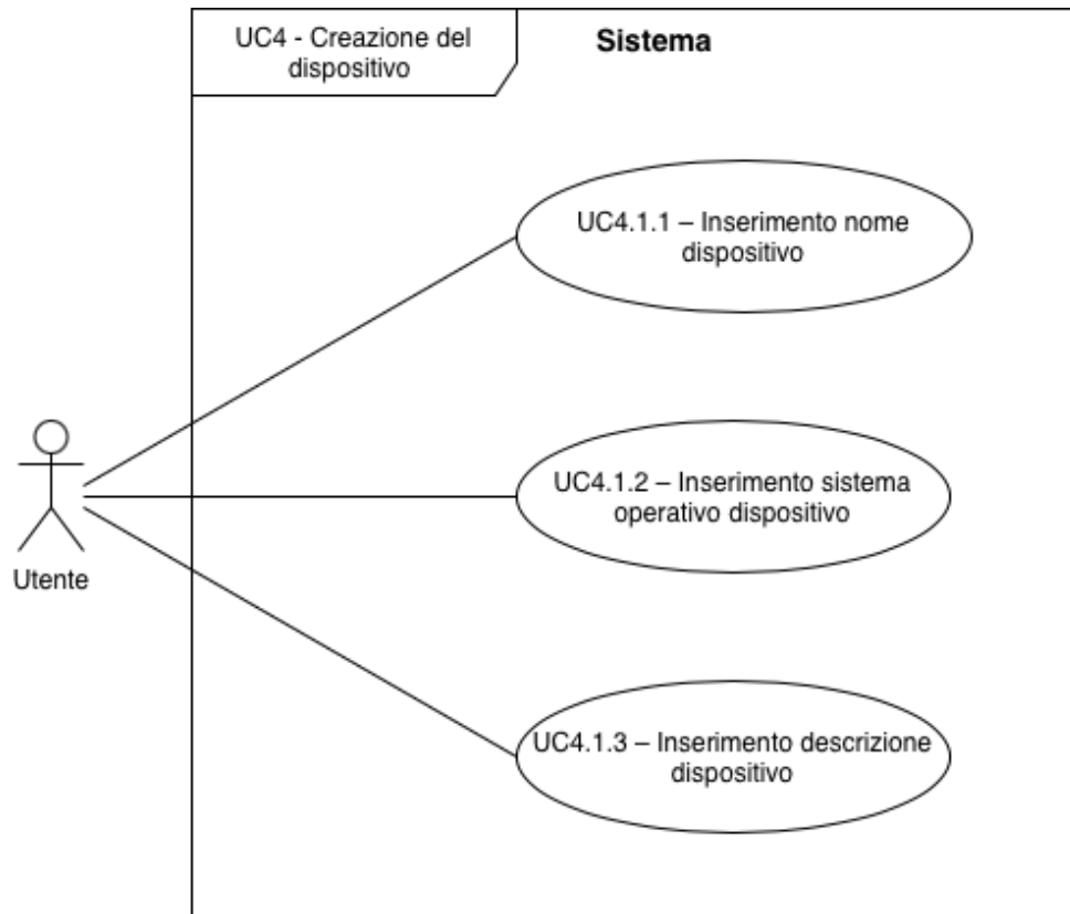
UC-4.1 : Inserimento nome, SO e descrizione dispositivo
