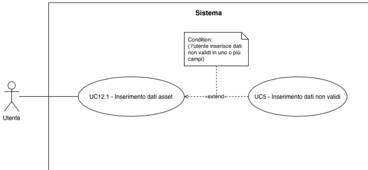
UC-12.1 : Inserimento dati asset G
