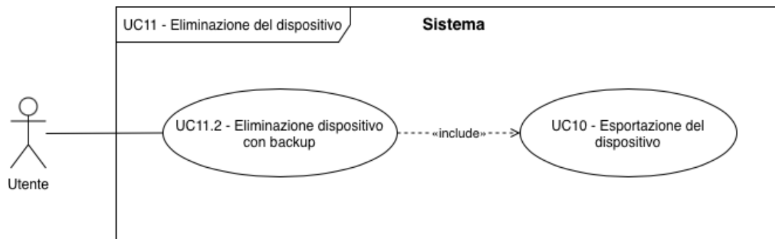
UC-11.2 : Eliminazione dispositivo con backup
