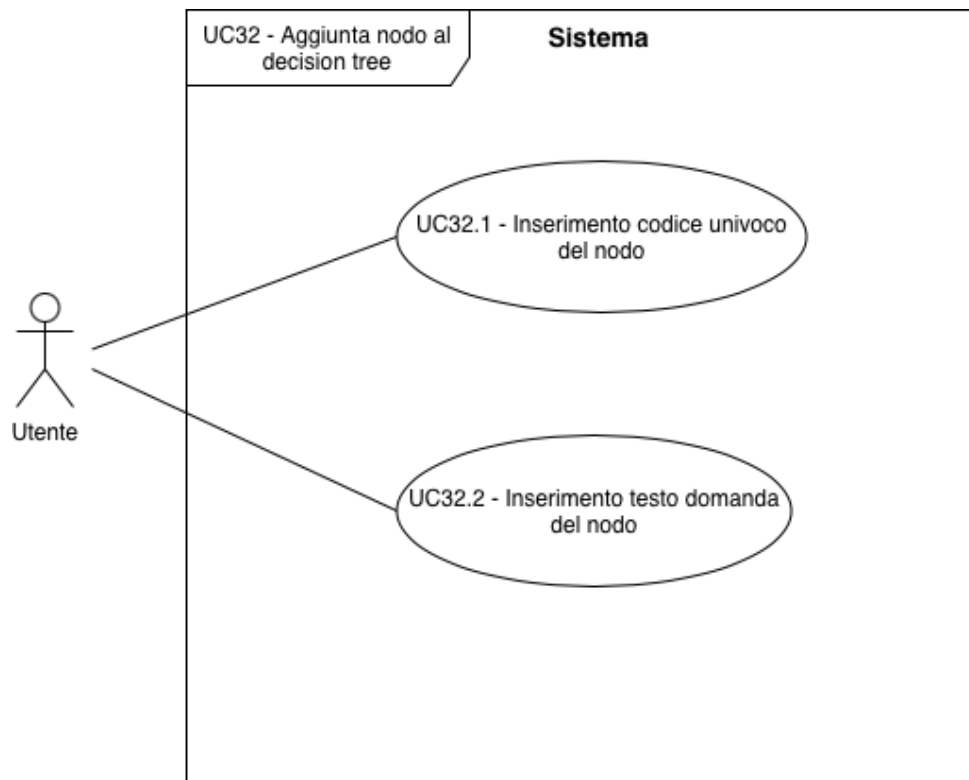
UC-32 : Inserimento codice e domanda del nodo
