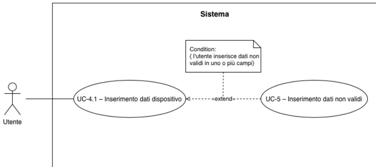
UC-4.1 : Inserimento dati dispositivo
