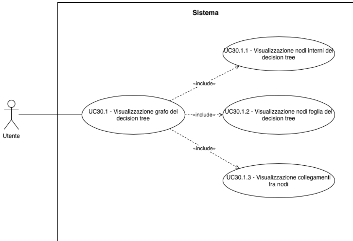
UC-30.1 : Visualizzazione grafo del decision tree G
