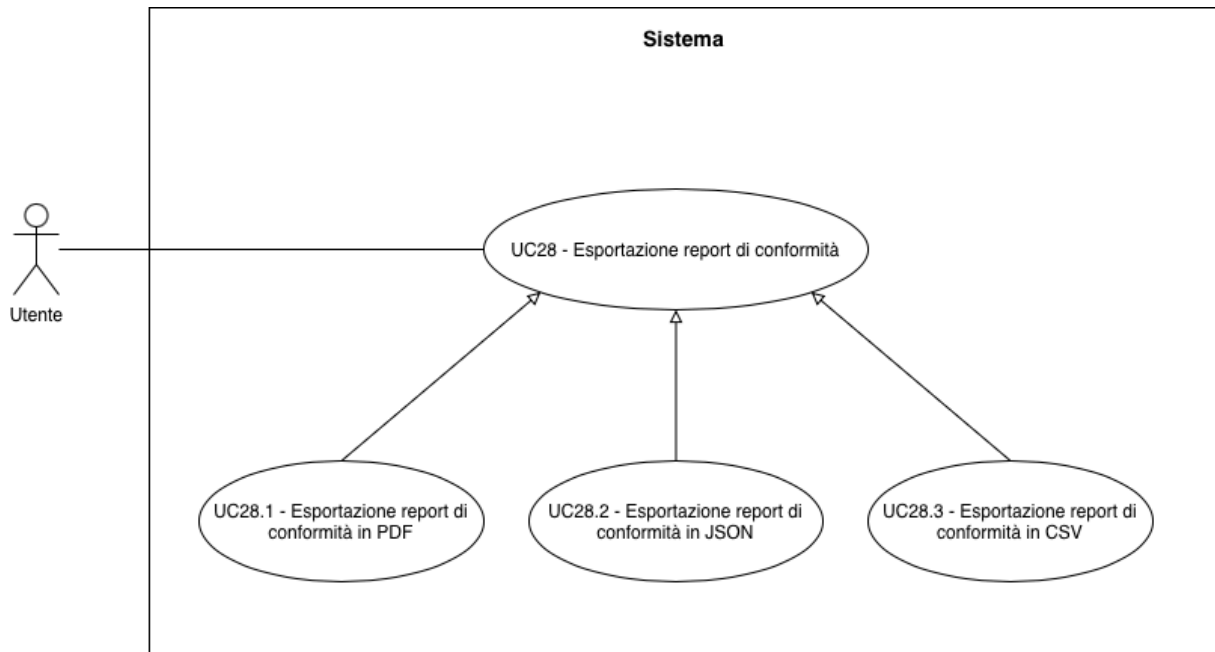
UC-28 : Esportazione report di conformità
