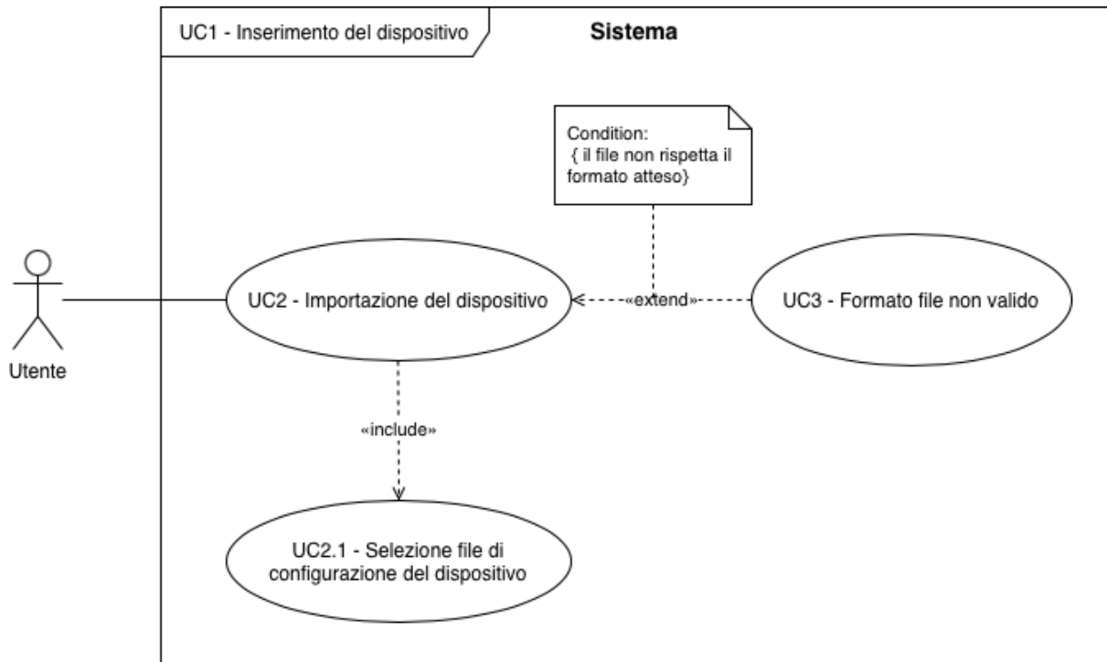
UC-2 : Importazione del dispositivo
