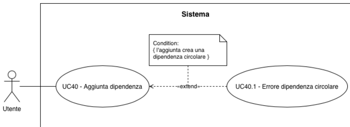
UC-40 : Aggiunta dipendenza
