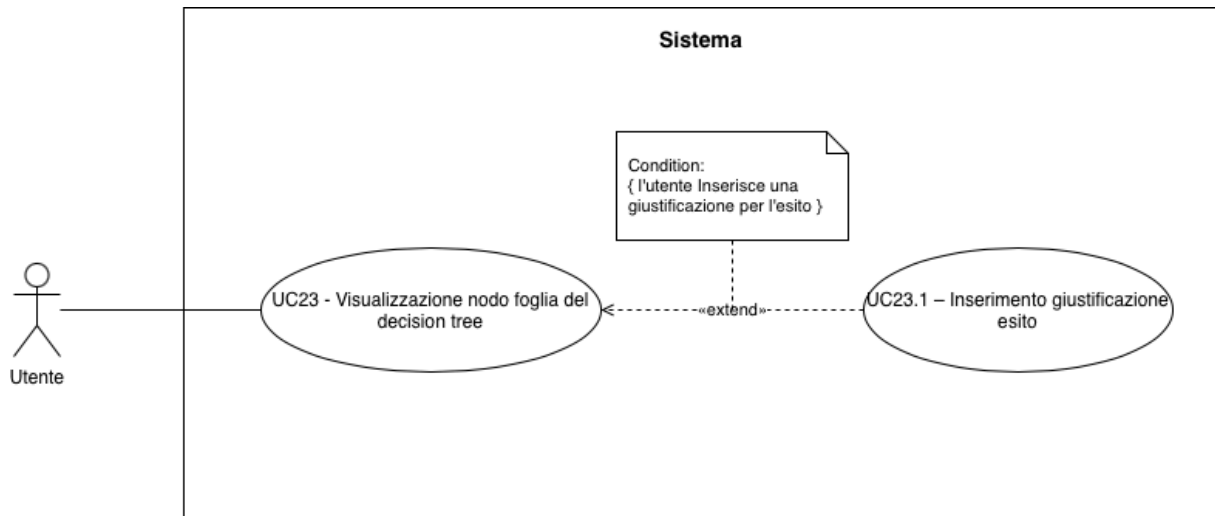
UC-23 : Visualizzazione nodo G foglia del decision tree G
