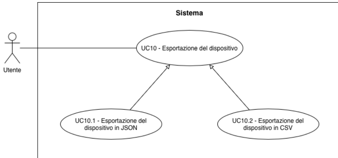
UC-10 : Esportazione del dispositivo
