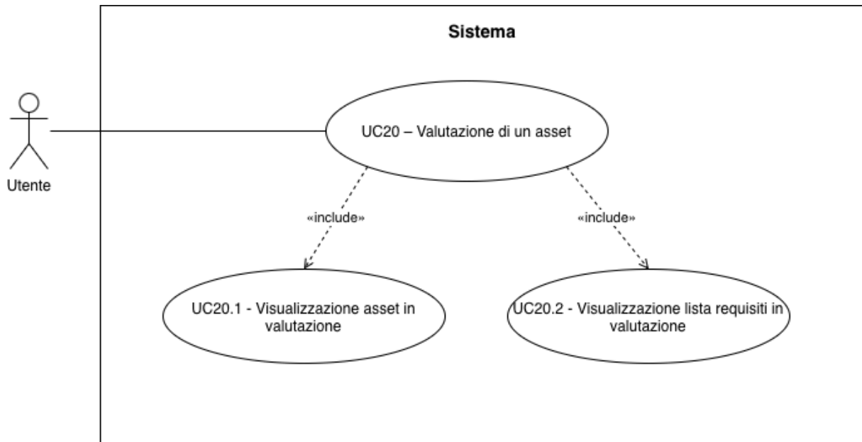
UC-20 : Valutazione di un asset G
