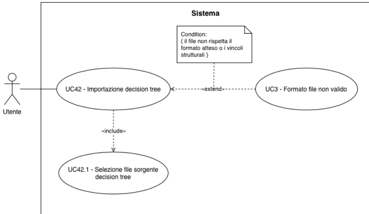
UC-42 : Importazione decision tree G
