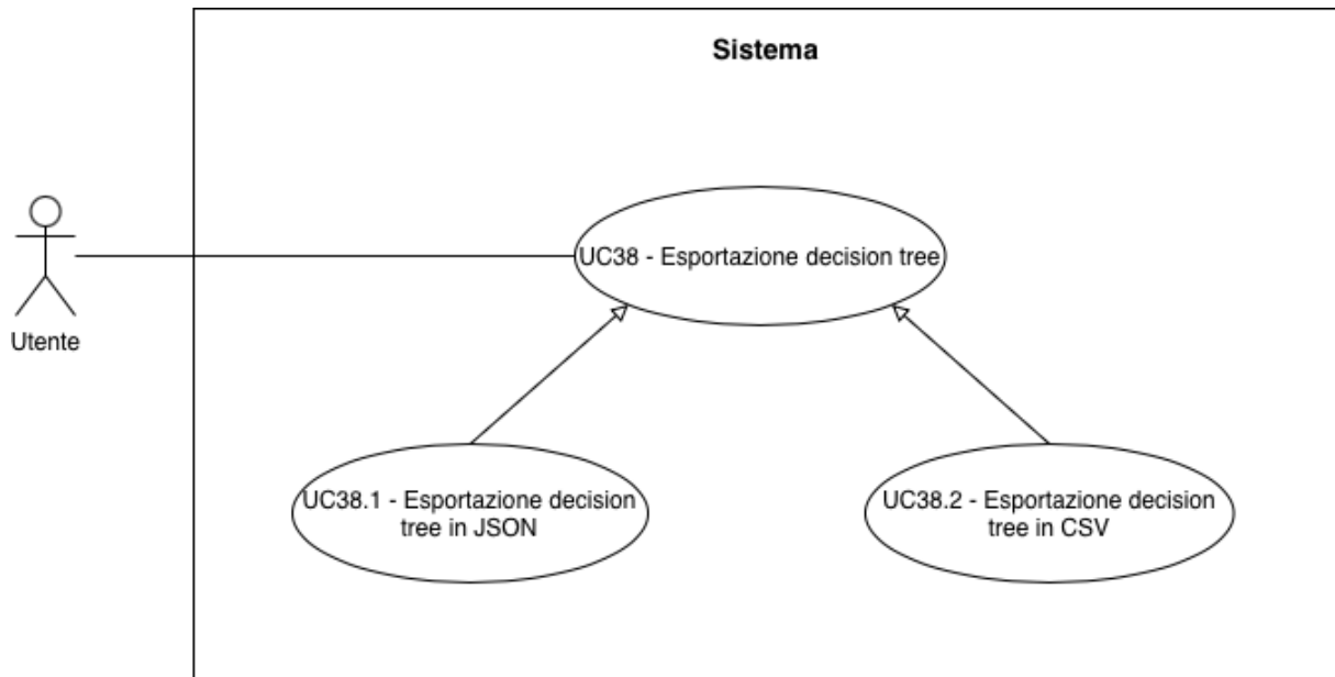
UC-38 : Esportazione decision tree G
