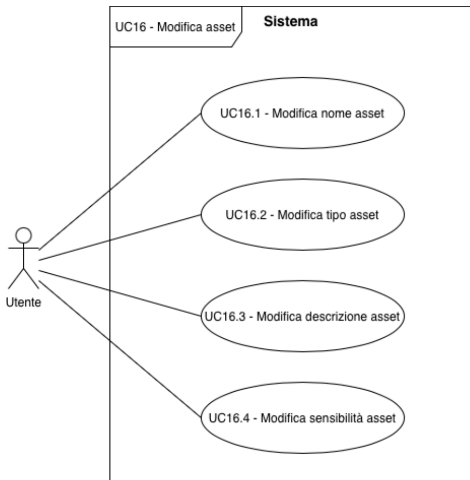
UC-16 : Modifica nome, tipo, descrizione e sensibilità asset G
