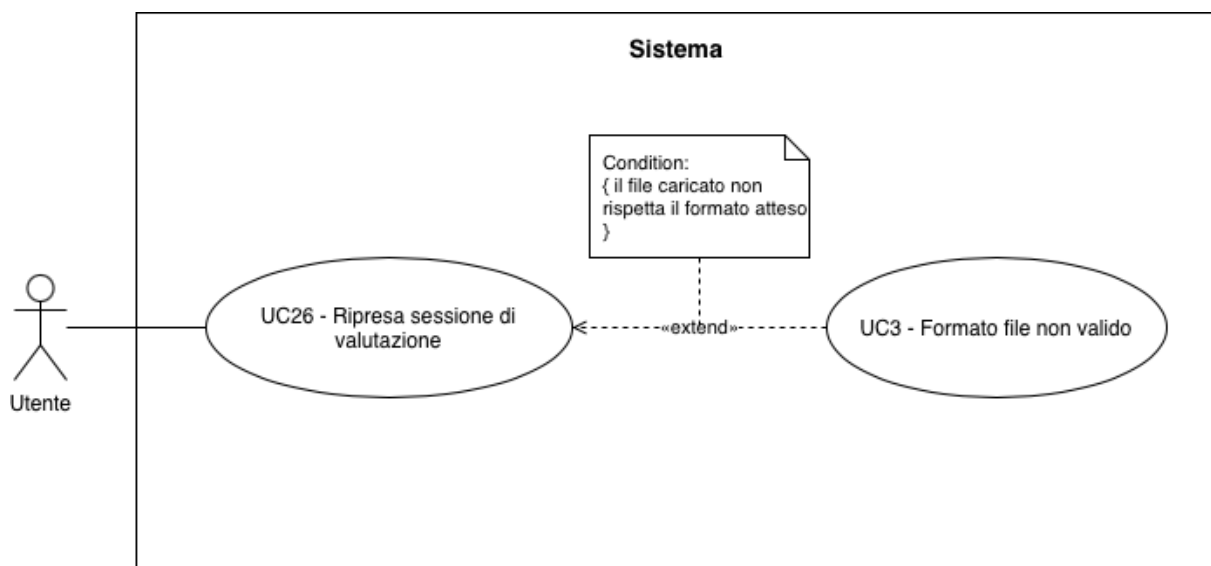
UC-26 : Ripresa sessione di valutazione
