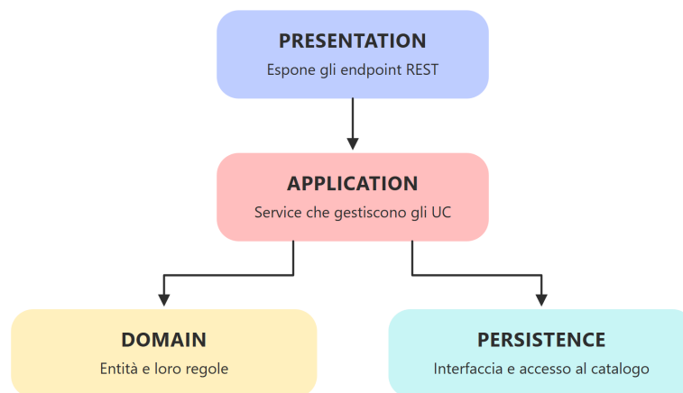
Figura 18: Backend G : i quattro livelli e la direzione delle dipendenze
