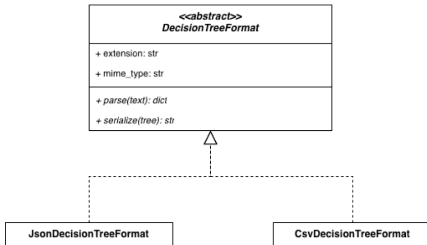
Figura 23: decision_tree_format: interfaccia G e realizzazioni
