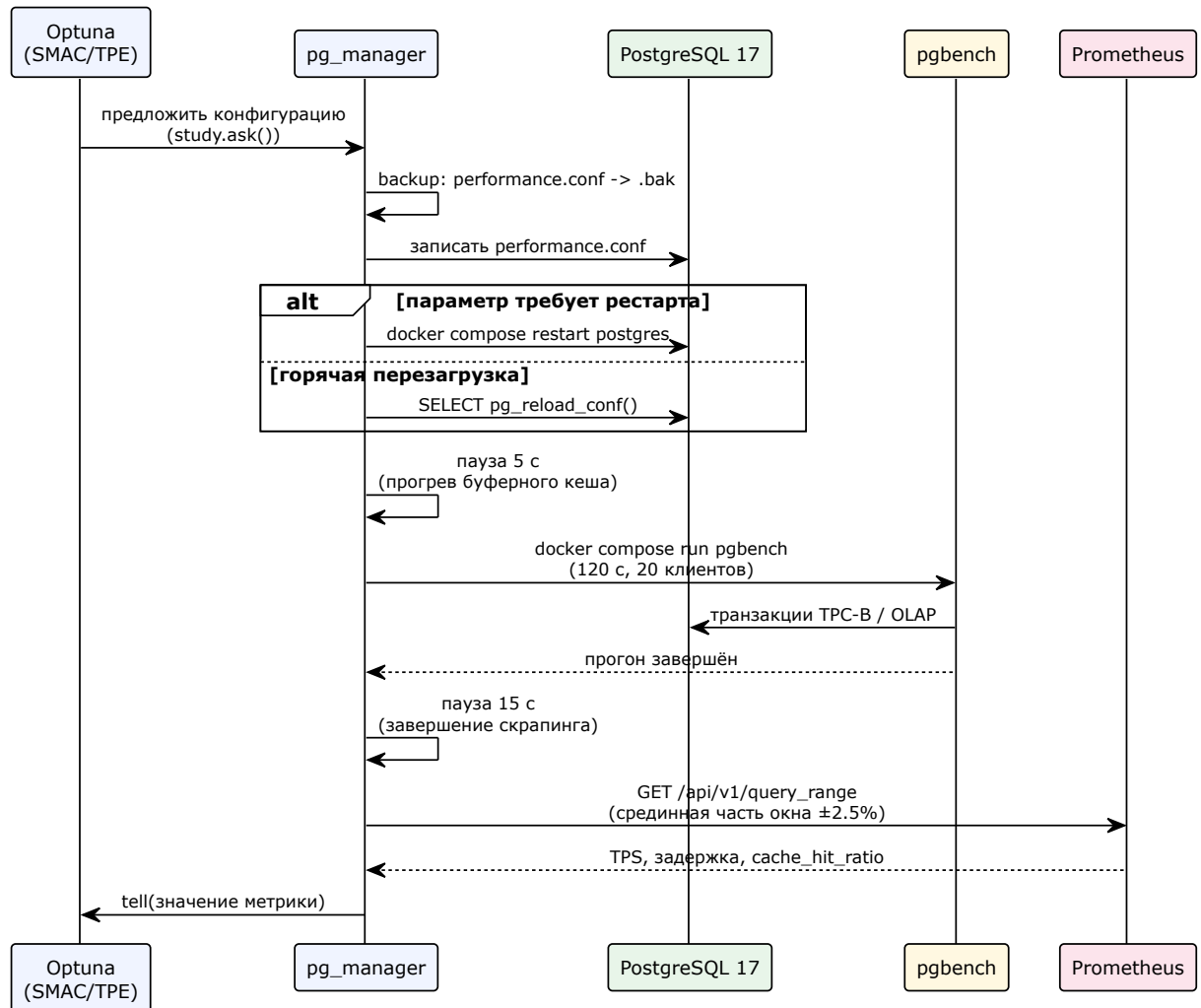
Рисунок 5 — Последовательность взаимодействия компонентов в рамках одной итерации оптимизации
