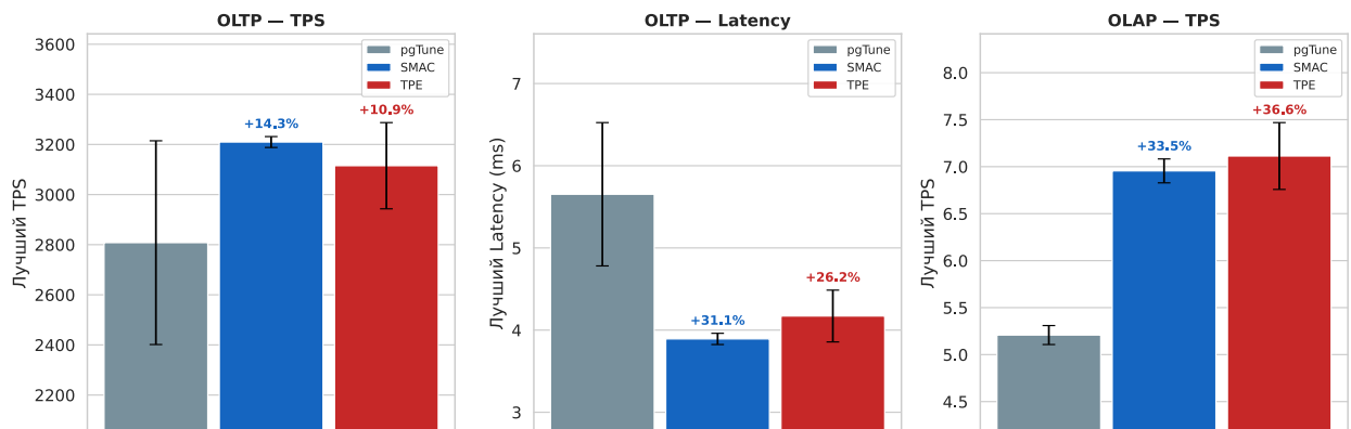
Рисунок 3 — Прирост производительности относительно pgTune (среднее \pm ст. откл., 3 запуска)
