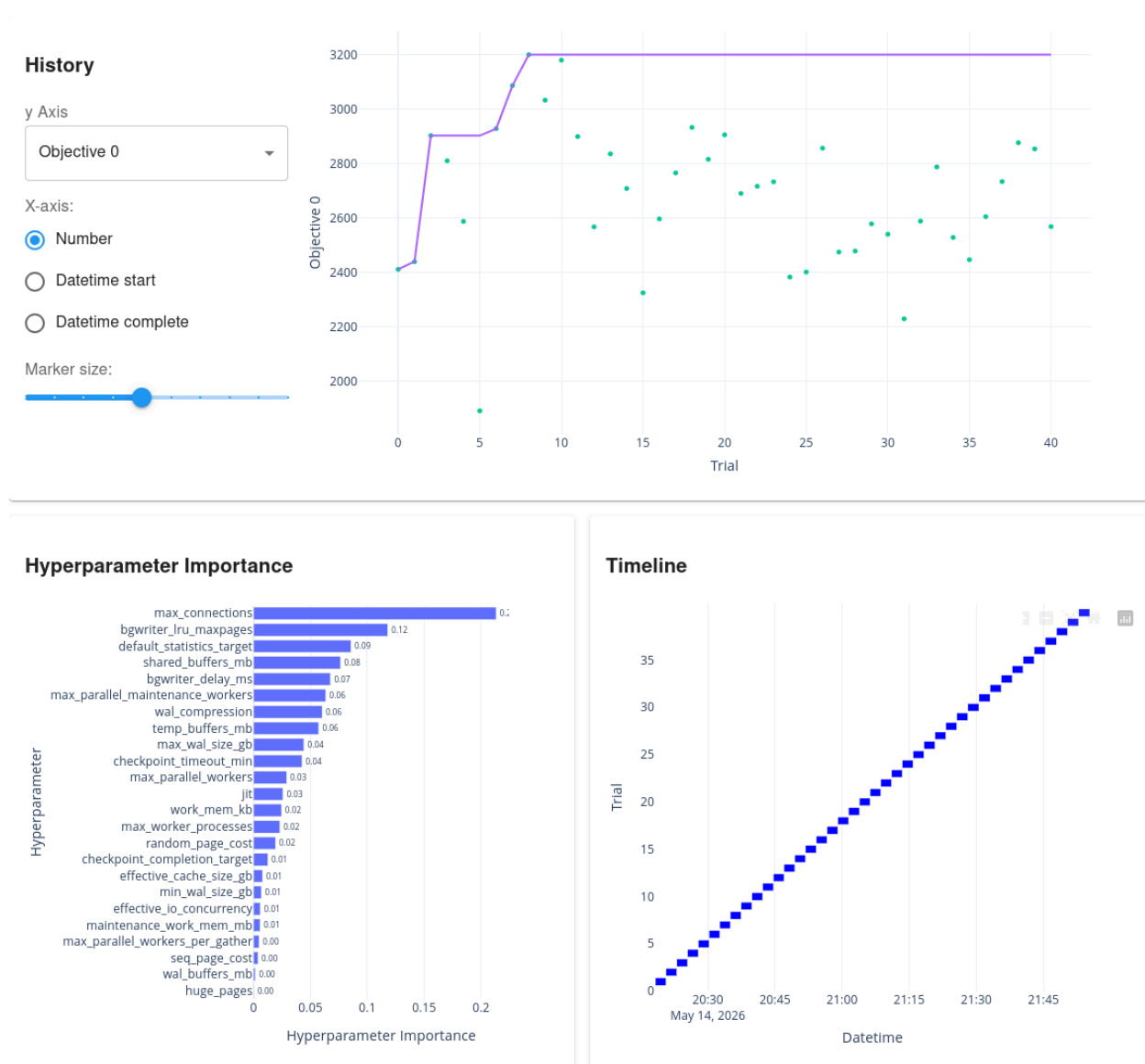
Рисунок 2 — Интерфейс optuna-dashboard для исследования pg_oltp_tps_smac_2026-05-14-20:13:34: история оптимизации, важность гиперпараметров и временная диаграмма прогонов
