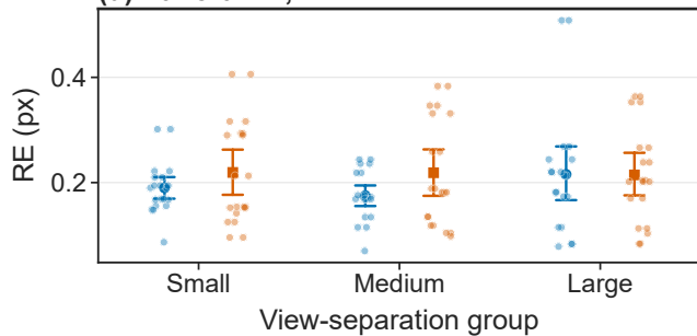
(d) Panoramix, RE
