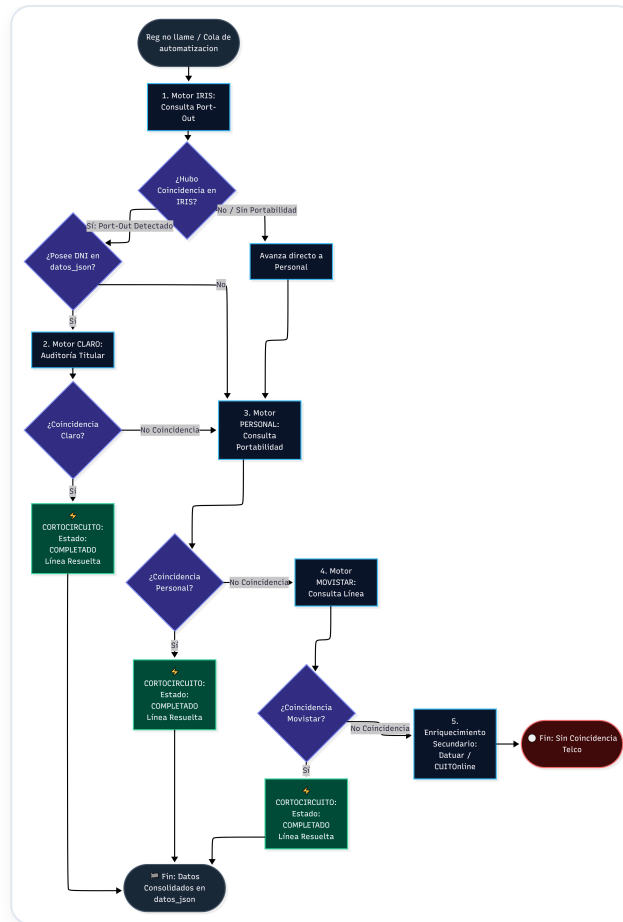
Diagrama 1 · Flujo de la cascada: IRIS → Claro → Personal → Movistar → enriquecimiento secundario (Datuar / CUITOnline). Los bloques verdes son cortocircuitos.
