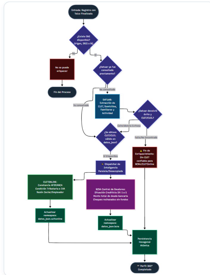
Diagrama 2 · Flujo de enriquecimiento: validación de DNI, Datuar, despacho paralelo a CUITOnline y BCRA, y persistencia atómica del Perfil 360°.
