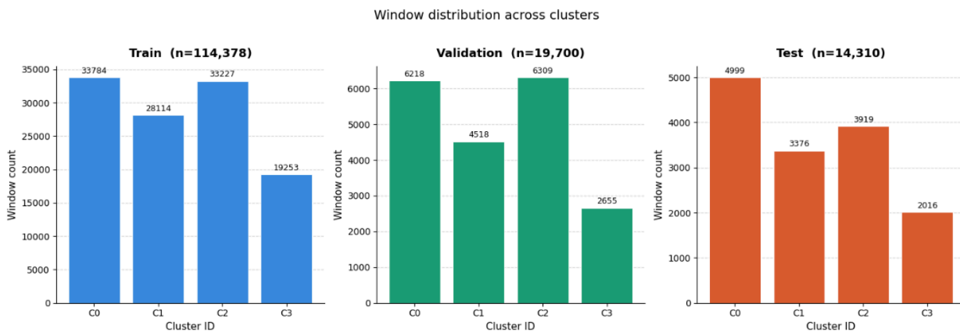
Figure 5: Распределение кластеров Handmade
