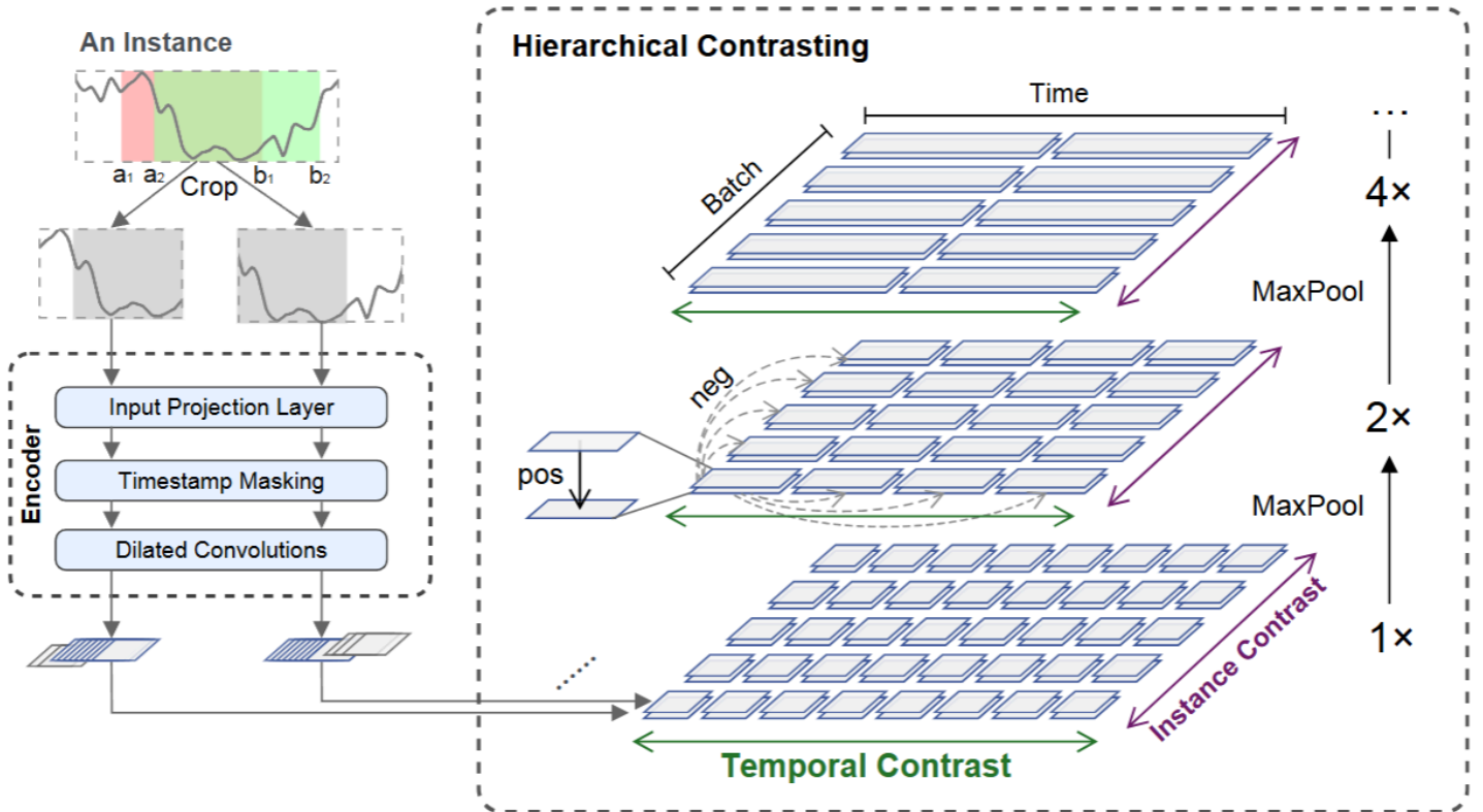
Figure 1: Схема архитектуры TS2Vec
