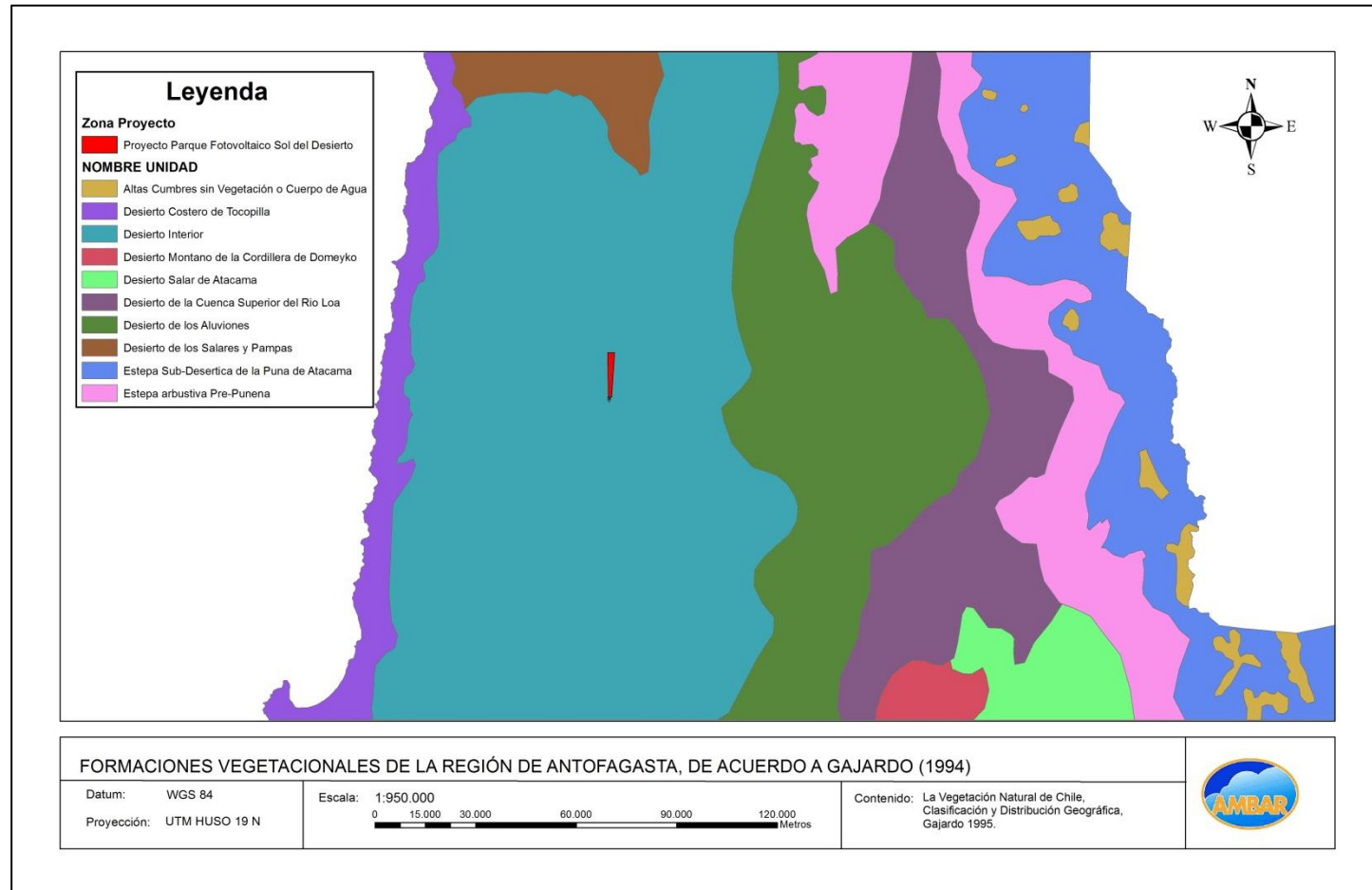
Figura 2. Formaciones vegetacionales de la región de Antofagasta de acuerdo a Gajardo (1994)
