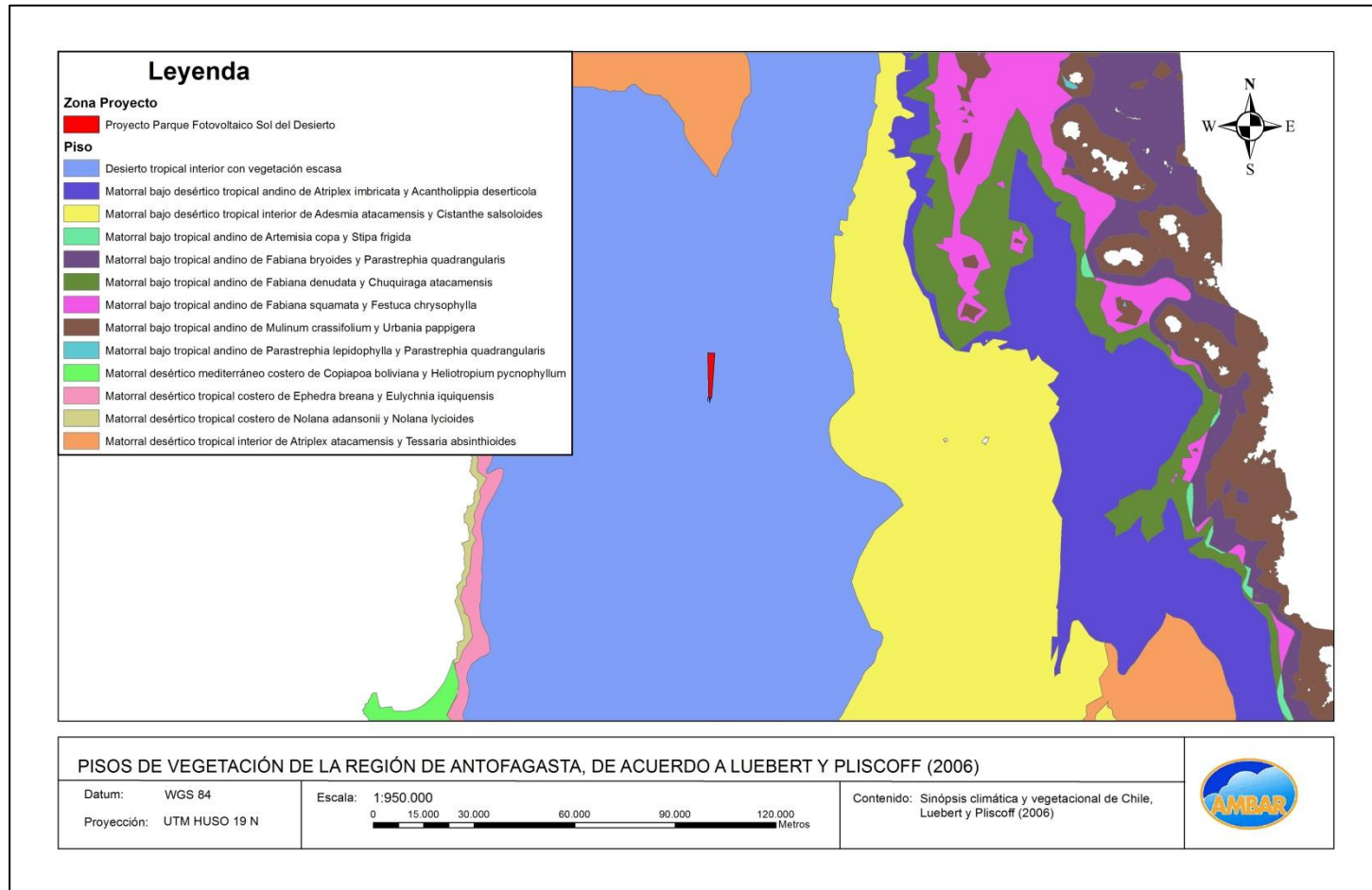
Figura 3. Pisos de vegetación de la región de Antofagasta de acuerdo a Luebert y Plischoff (2006)
