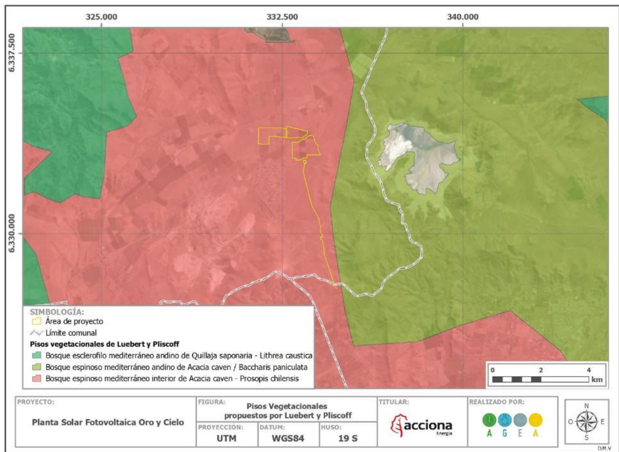
Figura 4-2: Ubicación del proyecto respecto a los pisos vegetacionales descritos por Luebert y Plischoff (2018)
