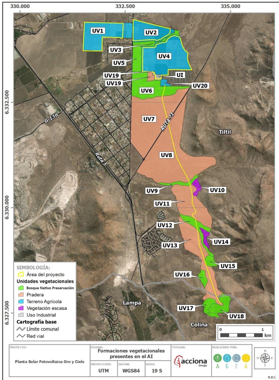
Figura 4-5 Formaciones vegetacionales presentes en el AI
