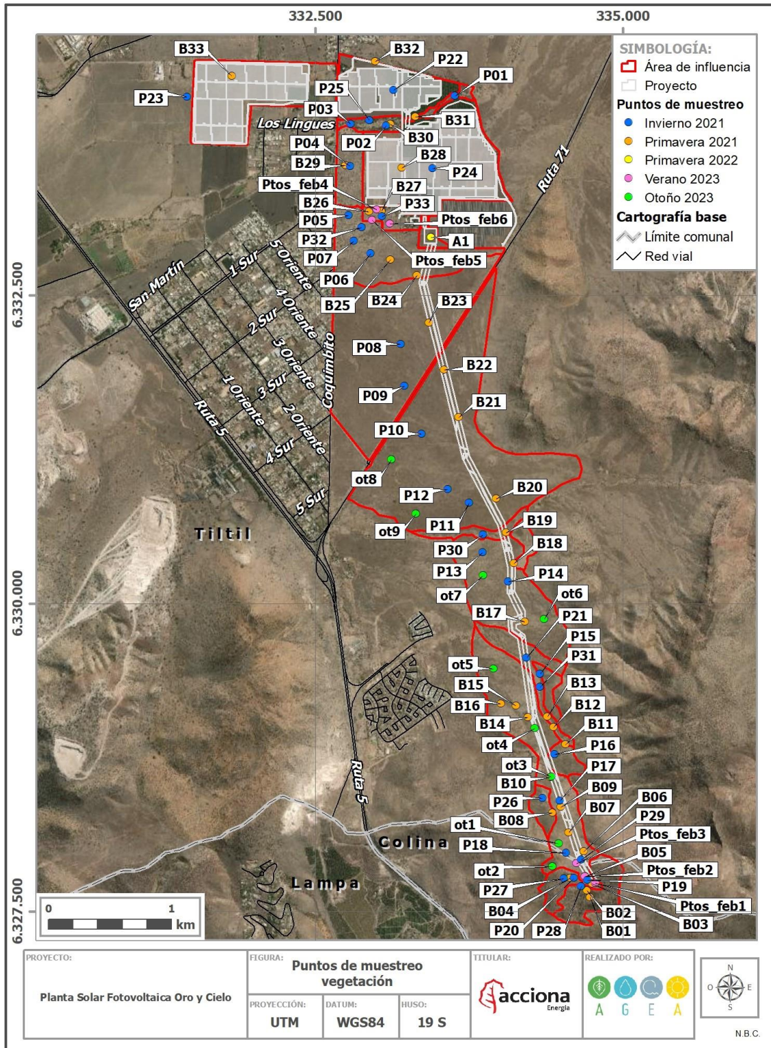
Figura 4-4: Puntos de muestreo
