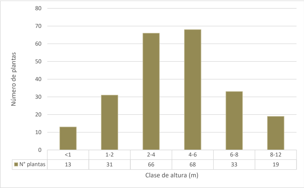
Gráfico 4-2 Número de algarrobos según clases de altura, sector Estero Peldehue
