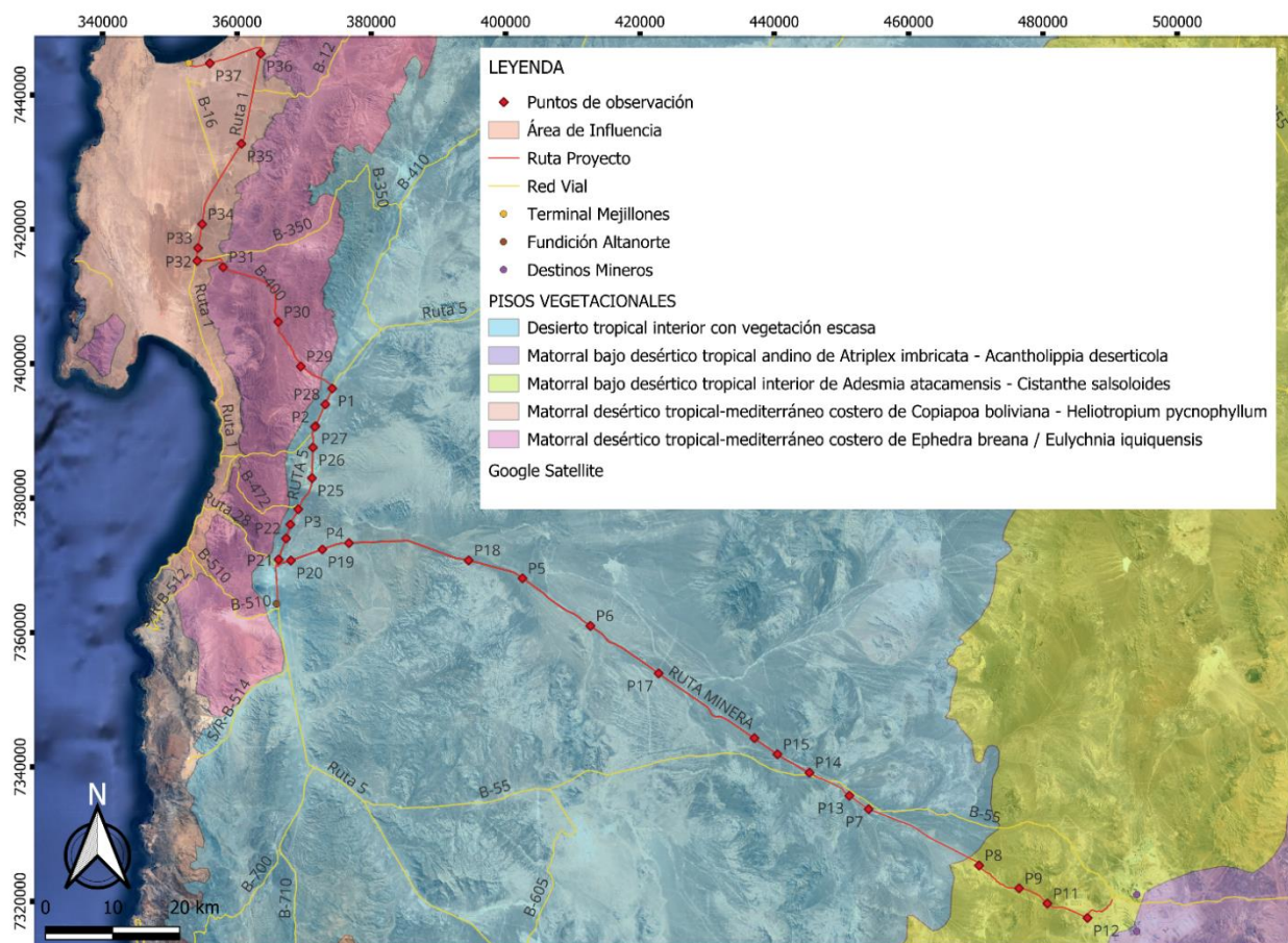
Figura 3. Pisos vegetacionales en el Área de Influencia del Proyecto (Luebert y Plischoff, 2017)
