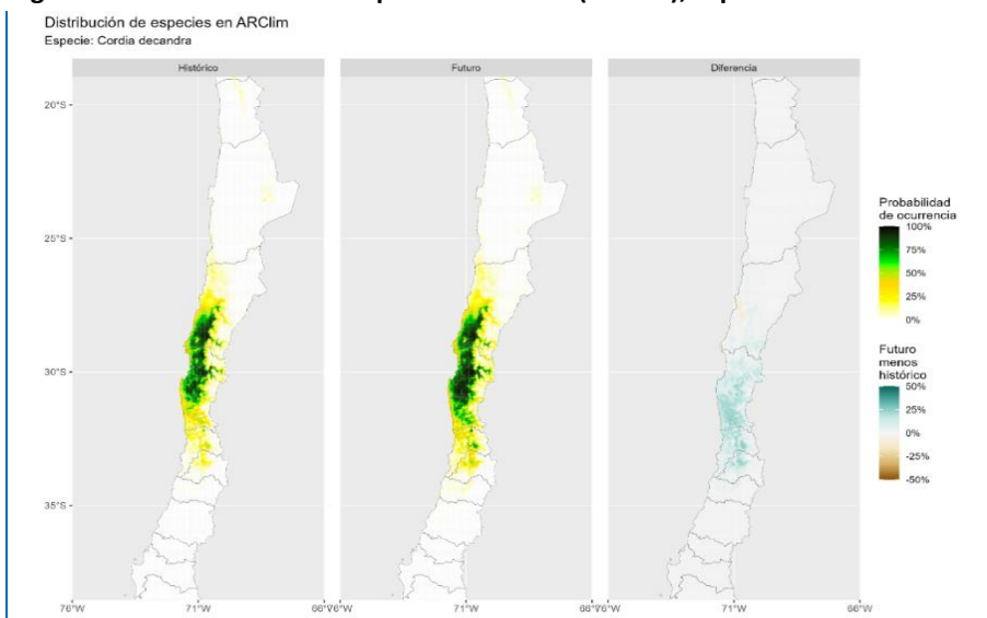
Figura 1-11. Distribución de especie en ARClím (detalle), Especie: Cordia decandra
