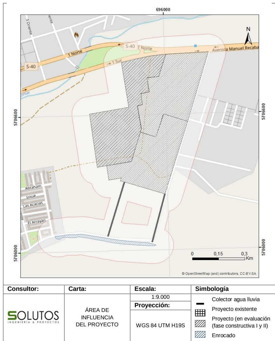
Figura 3. Área de Influencia del proyecto (AI).
