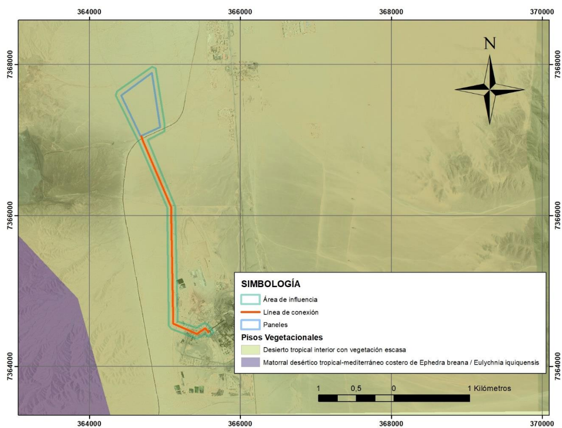
Figura 2. Pisos Vegetacionales de Luebert y Pliscoff identificados en el Área de Influencia.
