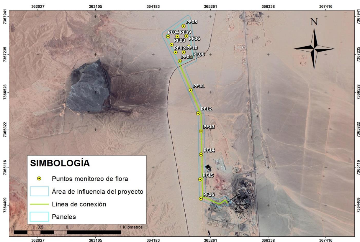
Figura 5. Puntos de Muestreo Flora en el Área de Influencia del Proyecto.
