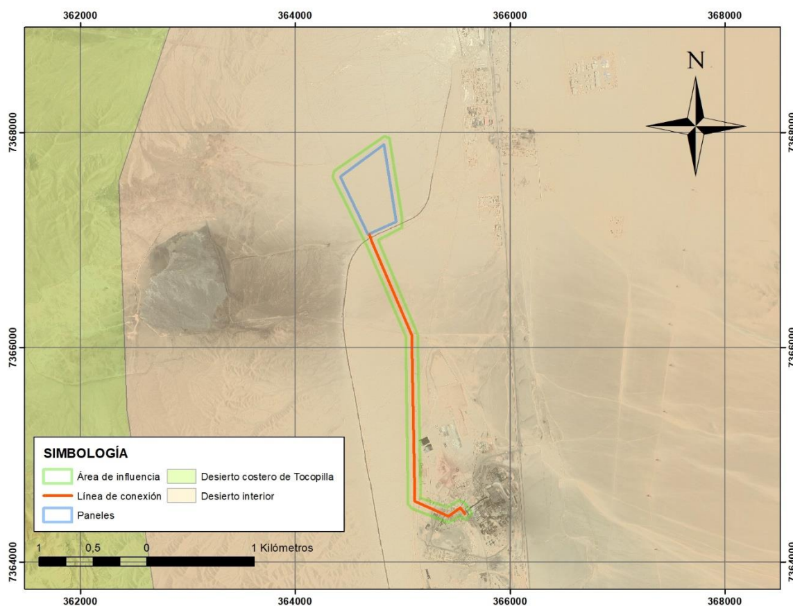
Figura 2. Área de influencia del proyecto en formaciones vegetacionales de Gajardo.
