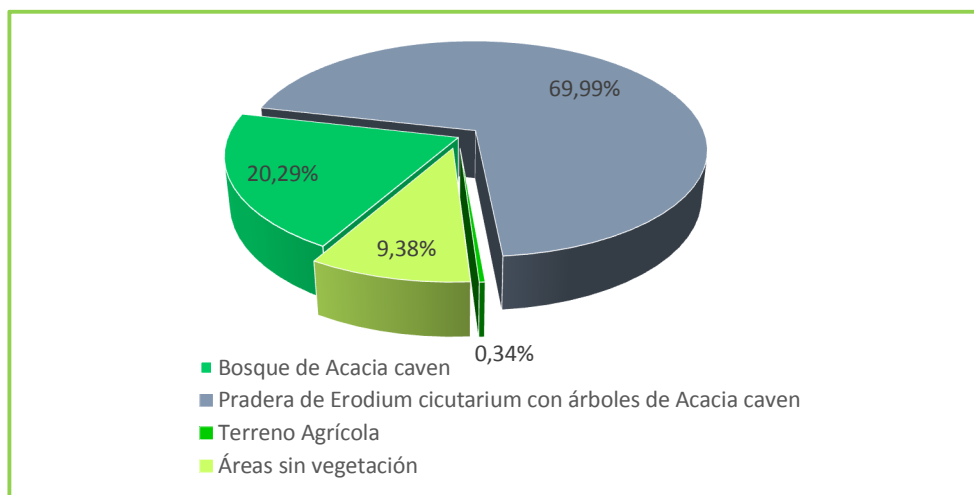
Figura 4. Representaciones Porcentuales de formaciones identificadas en el Área de Influencia.
