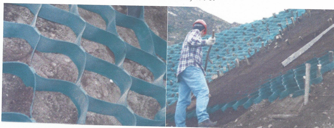
Figura A.5 Instalación malla Tenweb 300 y llenado de celdas
